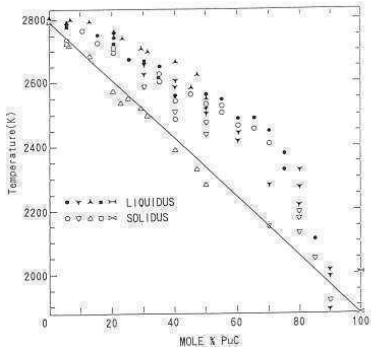
第 2.2.1 図 UC-PuC 系の融点
