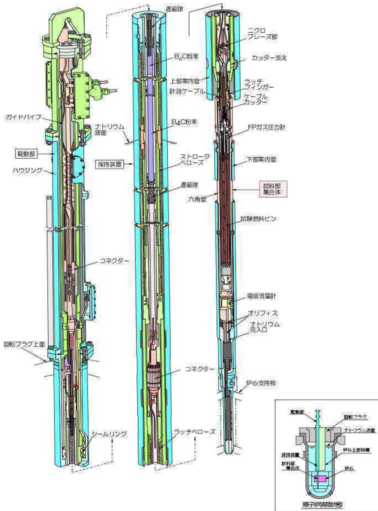
第5図 計測線付C型照射燃料集合体の構造
