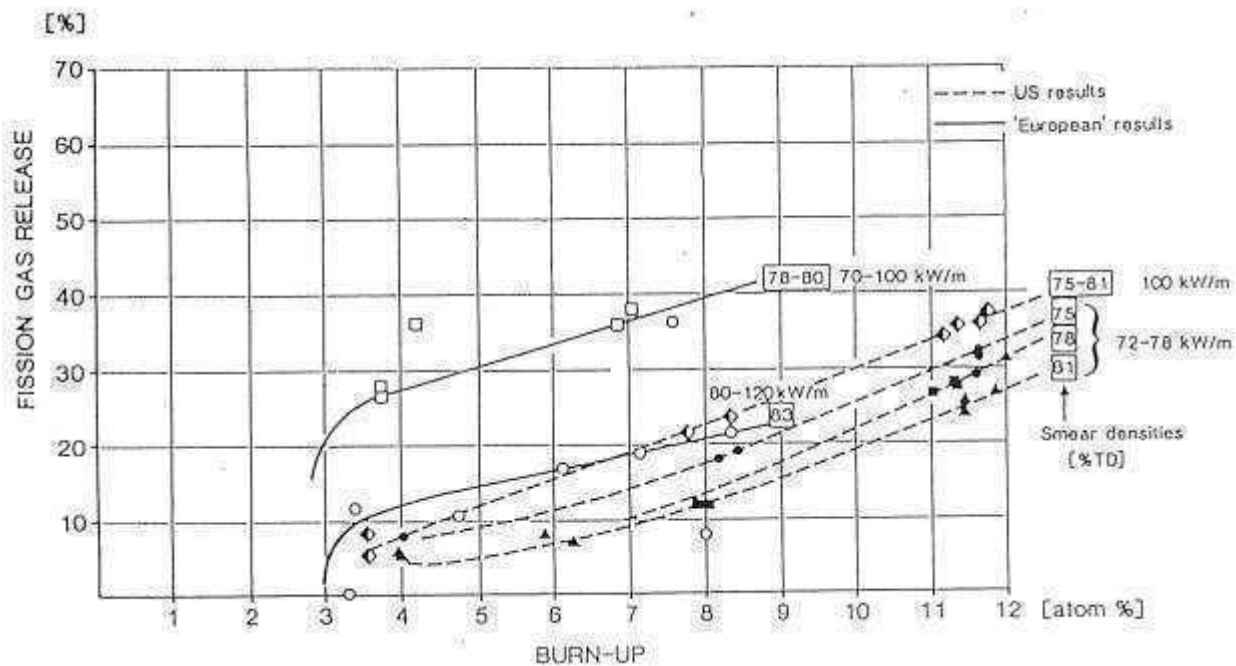
第2.4.1図 炭化物燃料のFPガス放出率
