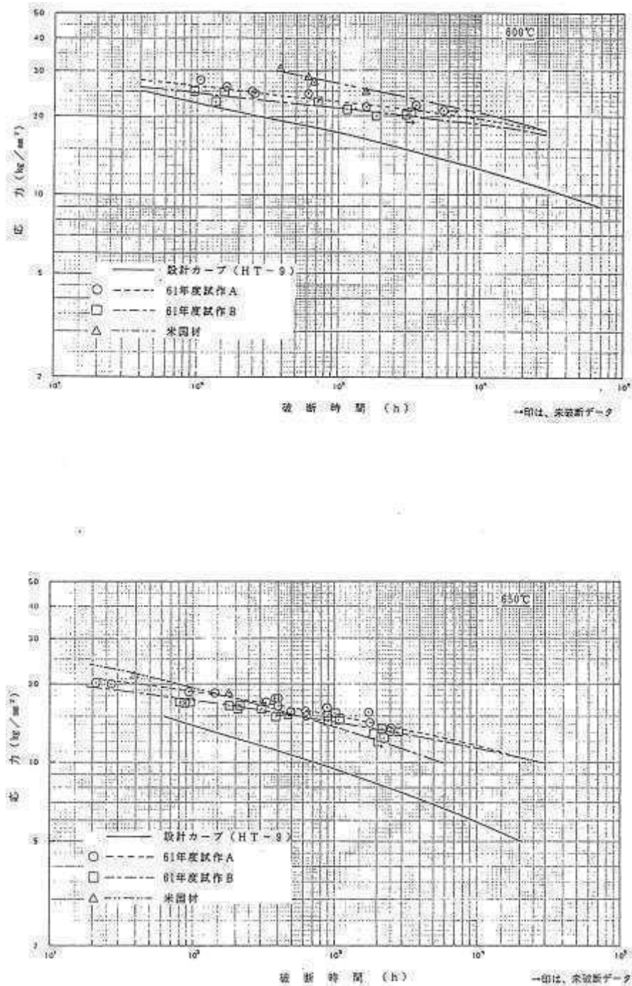
第 2.1.6 図 大気中クリープ破断強度
