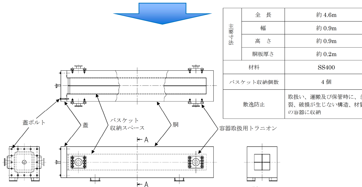
減容B P 運搬用容器概略図
