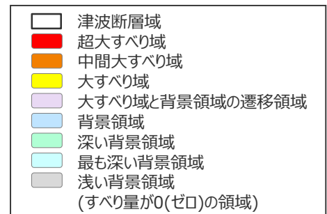
検討波源モデルB-1 (プレート境界面浅部・東海断層系) (大すべり域の位置を東へ10kmとしたケース)
