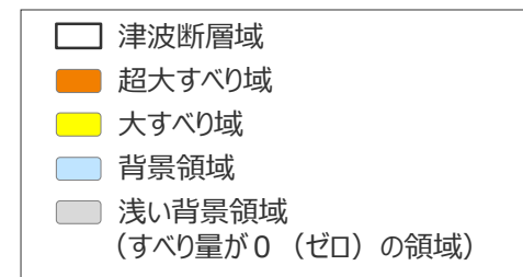
土木学会（2016）モデル
