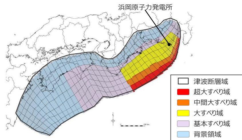
日本海溝の津波評価手法モデル③ (Δσ3.0MPa、RT150s)
