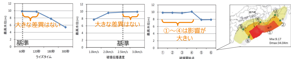
概略パラメータスタディの計算結果包絡値と津波痕跡高との比較
