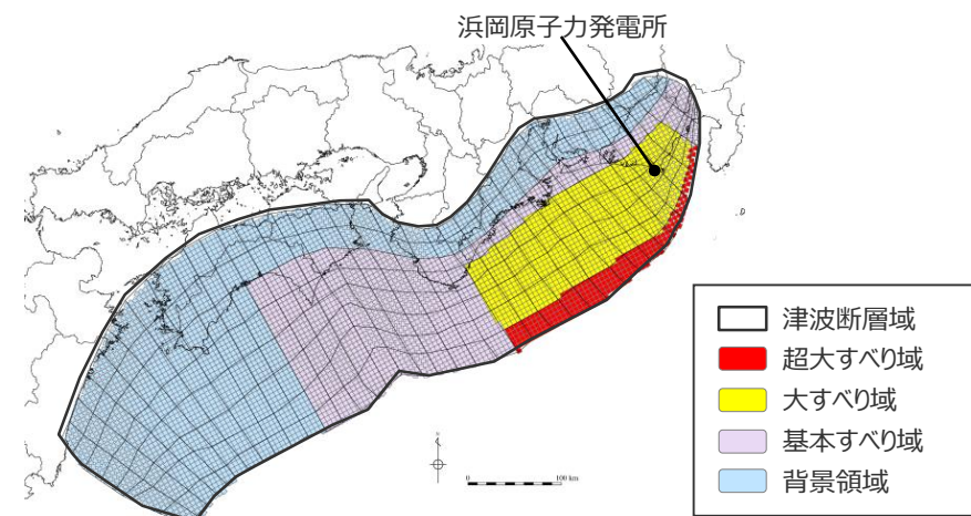
日本海溝の津波評価手法モデル② ( \Delta\sigma 3.0\text{MPa} 、RT150s)
