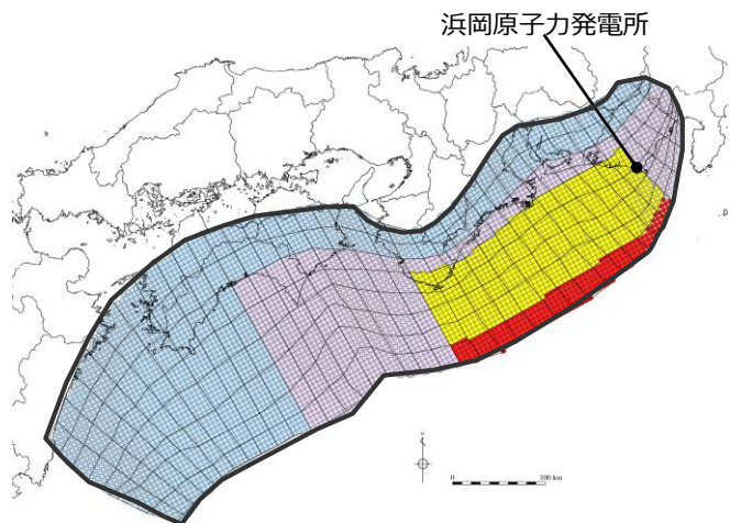
日本海溝の津波評価手法モデル②の大すべり域の位置を西へ40kmとしたケース
