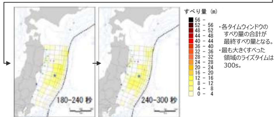
(内閣府(2012)を基に作成)
