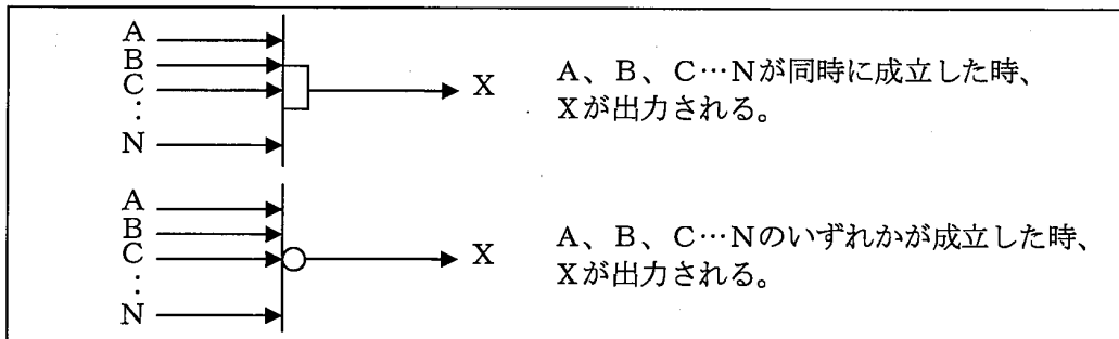
図-67 (1/2) 脱水ろ液タンク液面異常高による受入れ停止のインターロック
