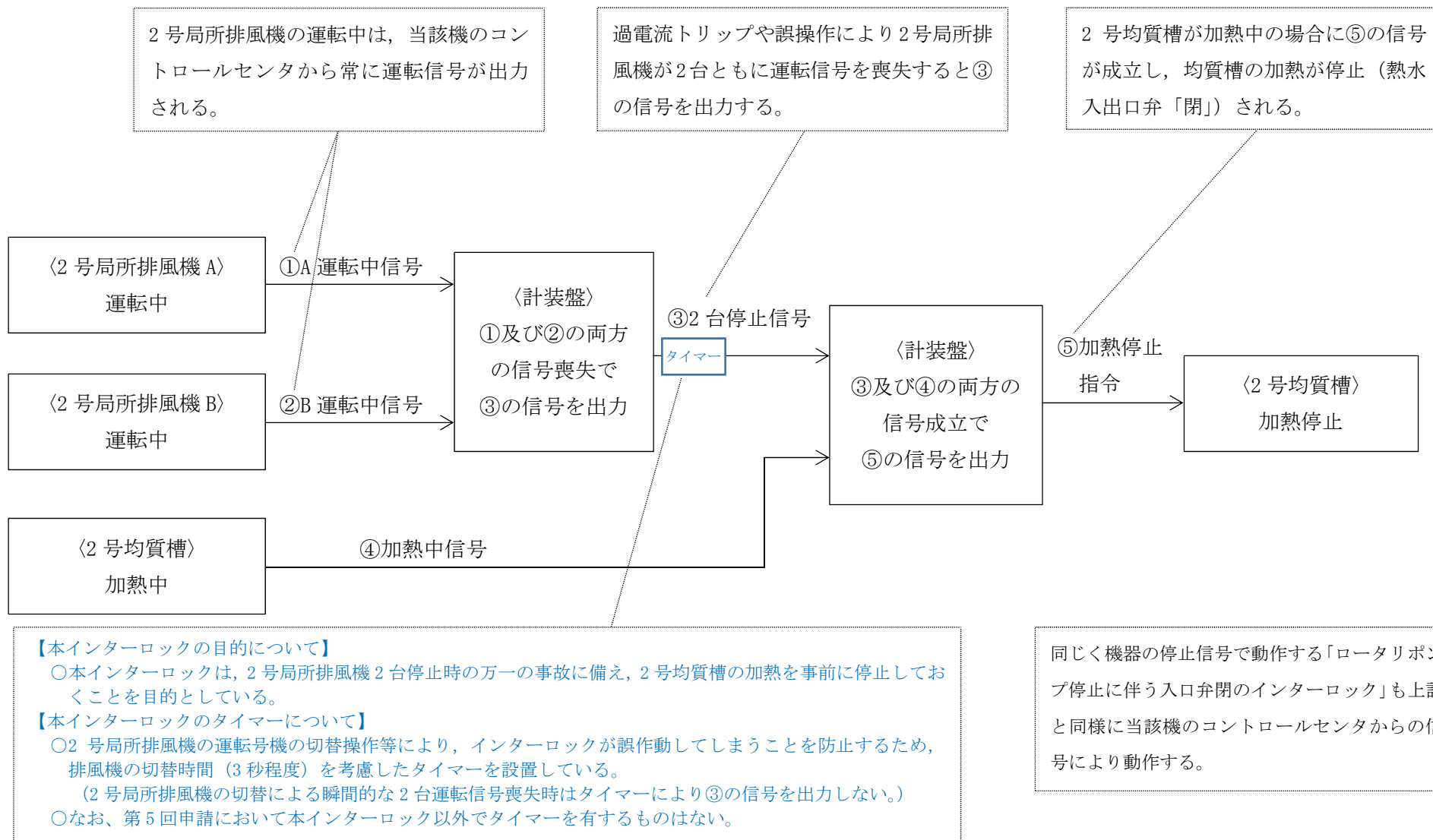
機器の停止信号で動作するインターロックの信号の流れの概要図 (2号局所排風機2台停止による加熱停止インターロックの例)
