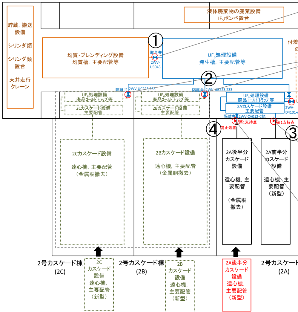
図1 各申請における設備の配管の取合いについて
