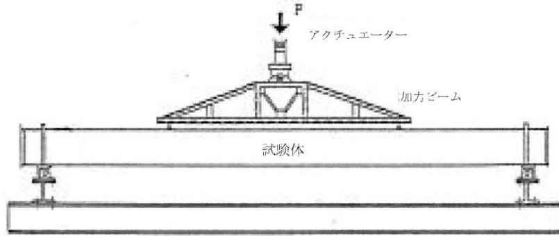
図 2-1 試験装置概要図
