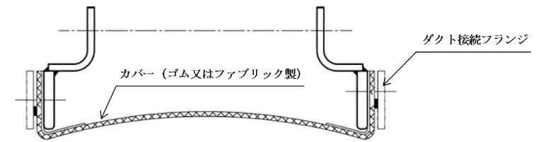
フレクター (断面図)
