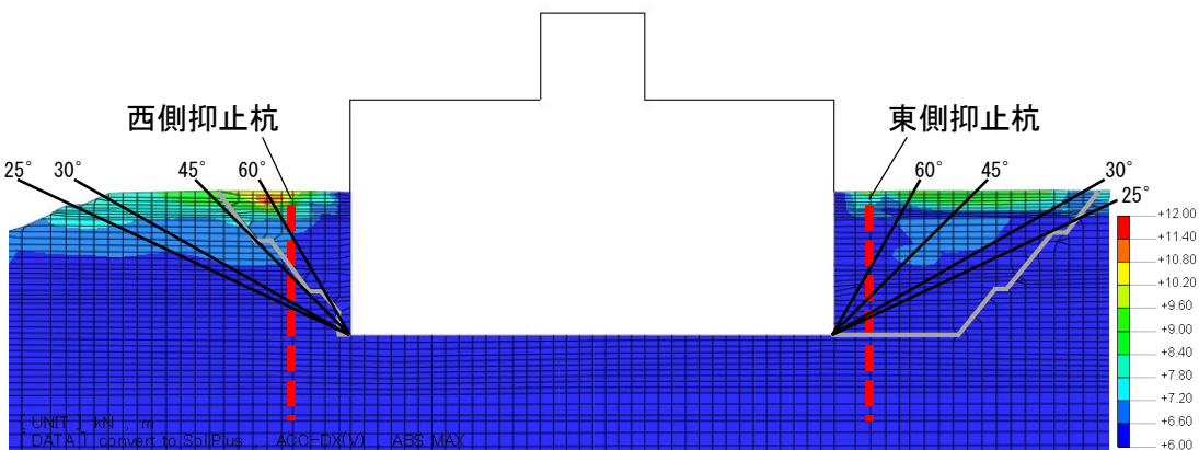
最大加速度 (水平成分) (m/s 2 )
