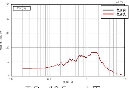
T.P.+18.5 m: 水平
