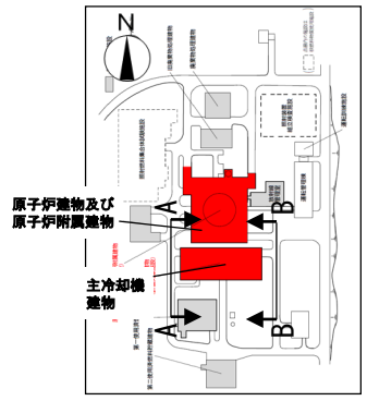
施設配置図
