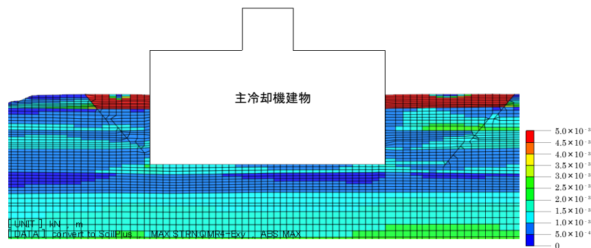
最大せん断ひずみ (—)
