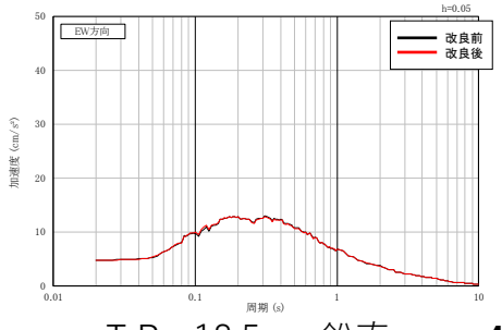
T.P.+18.5 m: 鉛直
