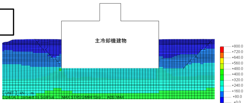
最大せん断応力 (kN/m 2 )
