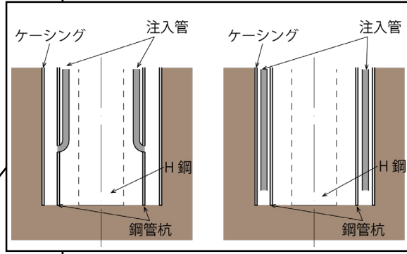
モルタル充填方法の例
