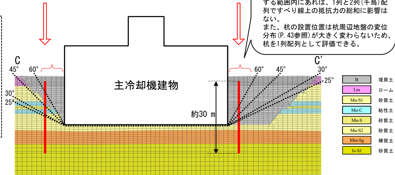
図 抑止杭周辺拡大図 (C-C' 断面)
