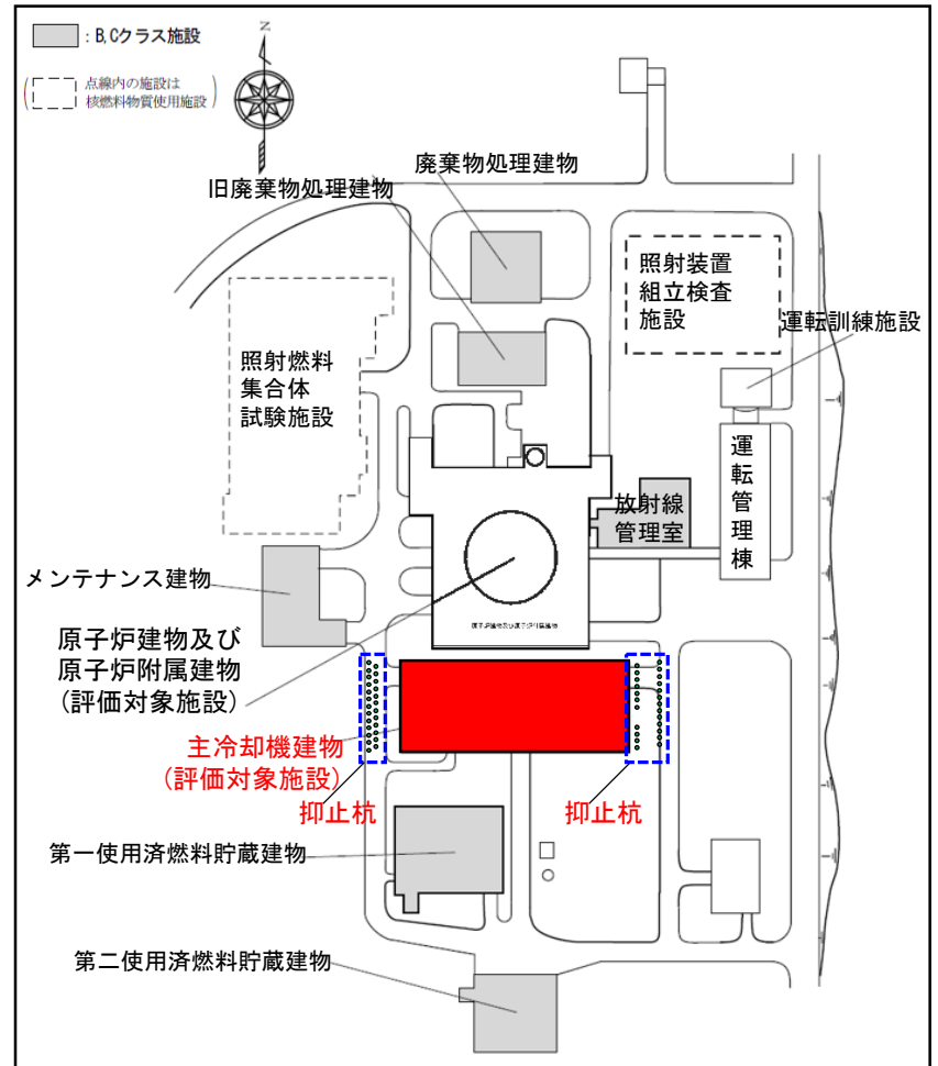
図 施設配置図
