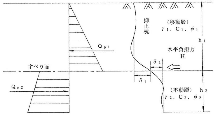
図 抑止杭に作用する受働土圧(最新斜面・土留め技術総覧より抜粋)
