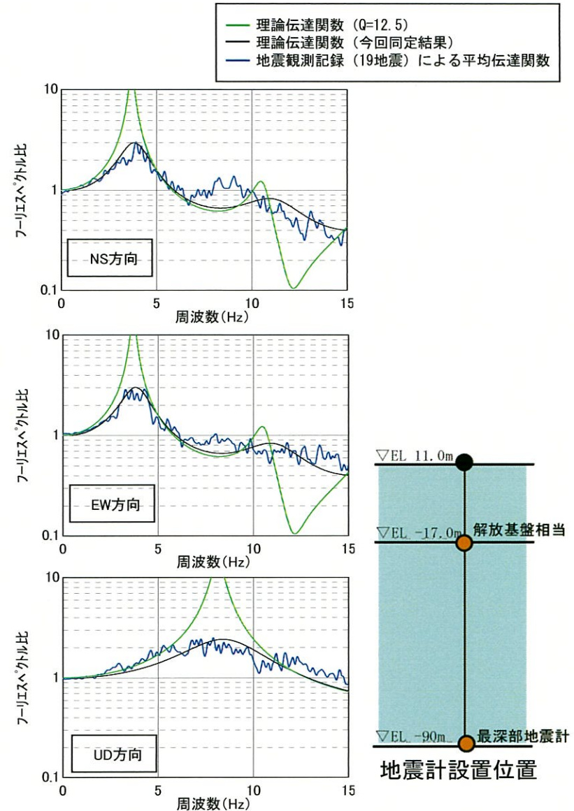
伝達関数の比較 (EL. -17m/EL. -90m)
