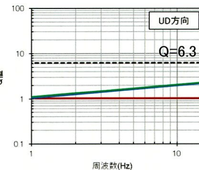
伝達関数により同定された地盤減衰(EL.+11m~EL.-90m)
