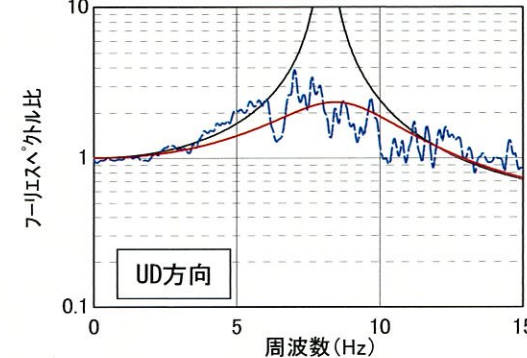
伝達関数 (EL. -17m/EL. -90m) の比較
