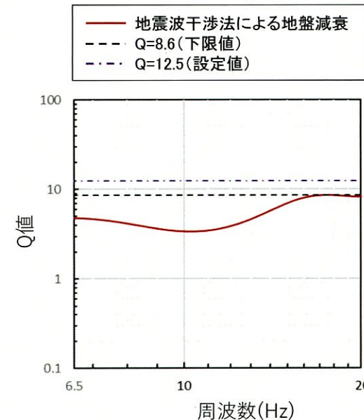
地震波干渉法により推定された地盤減衰(EL.+11m~EL.-90m)
