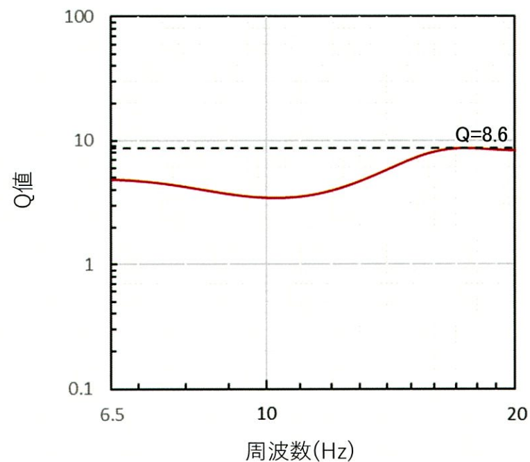
地震波干渉法により推定された地盤減衰 (EL.11m~EL.-90m)
