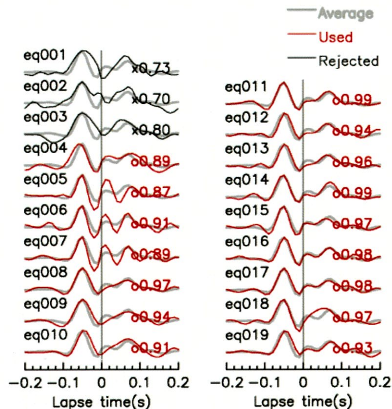
全地震の波形の平均と各地震の波形の相関
