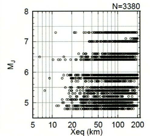
Xeq-Mjの分布
