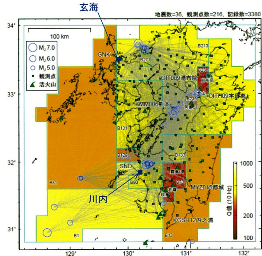
検討に用いた地震の震央分布及び観測点位置
