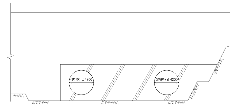
③~③断面 (図 3-9)
