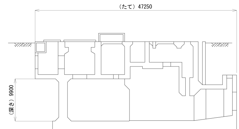
A~A 断面
