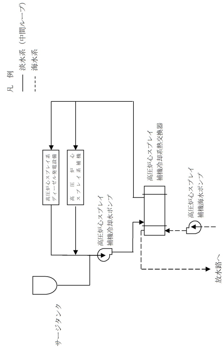
図 3-8 高圧炉心スプレイ補機冷却系 (高圧炉心スプレイ補機海水系含む。) 系統概要図
