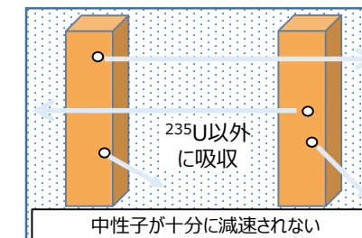
低水密度領域 での中性子挙動 （③）
