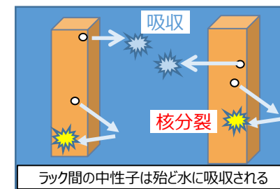
高水密度領域 での中性子挙動 （①）
