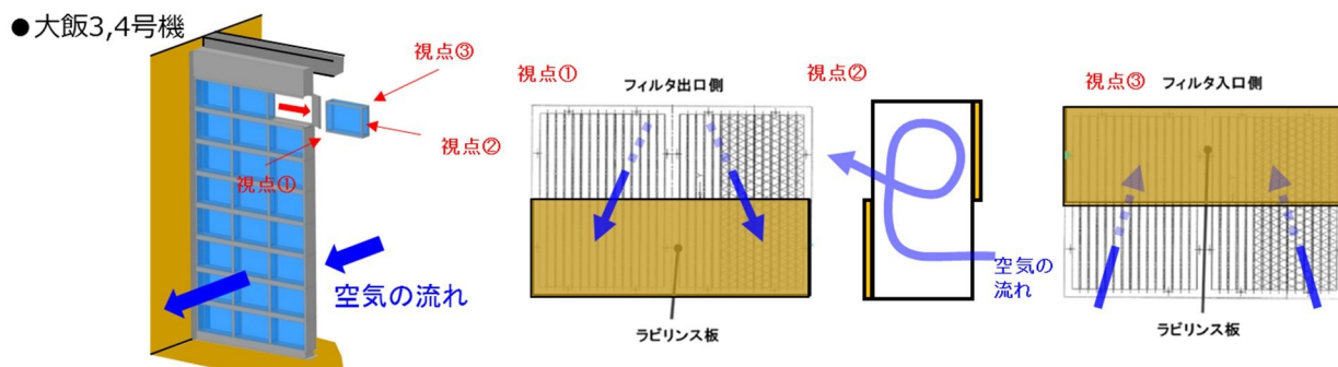
図1 改良型フィルタのラビリス板取付け状況
