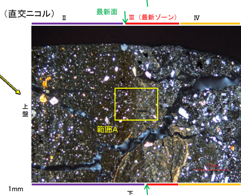
観察用薄片写真(E-8.60_126R)(拡大)
