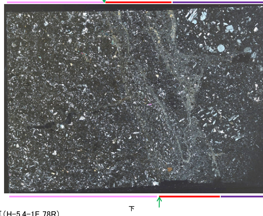
観察用薄片写真(H-5.4-1E_78R)
