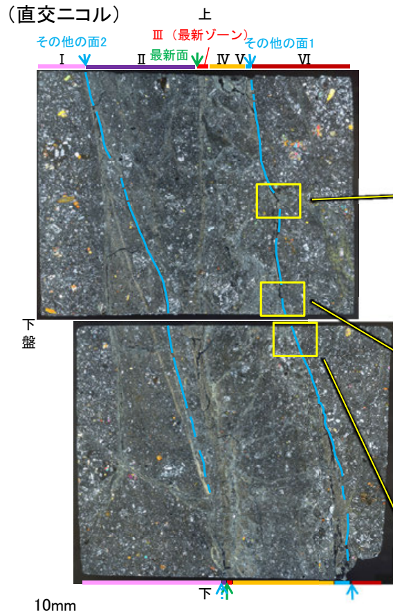
薄片写真(解釈線あり) (上:薄片② 下:薄片①)
