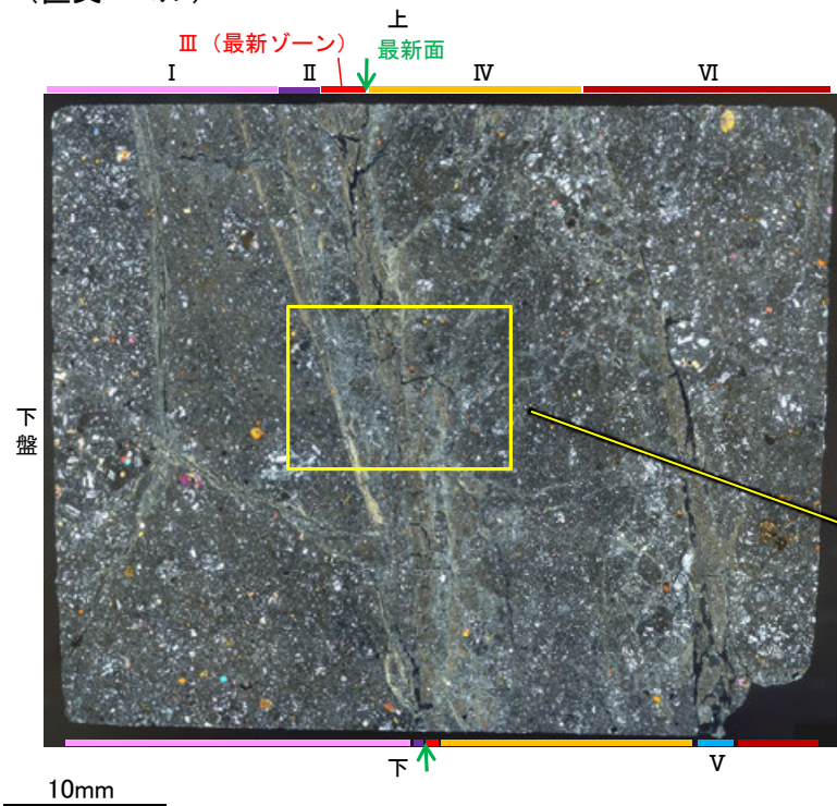
薄片①写真(R-8.1-1-3_109R)
