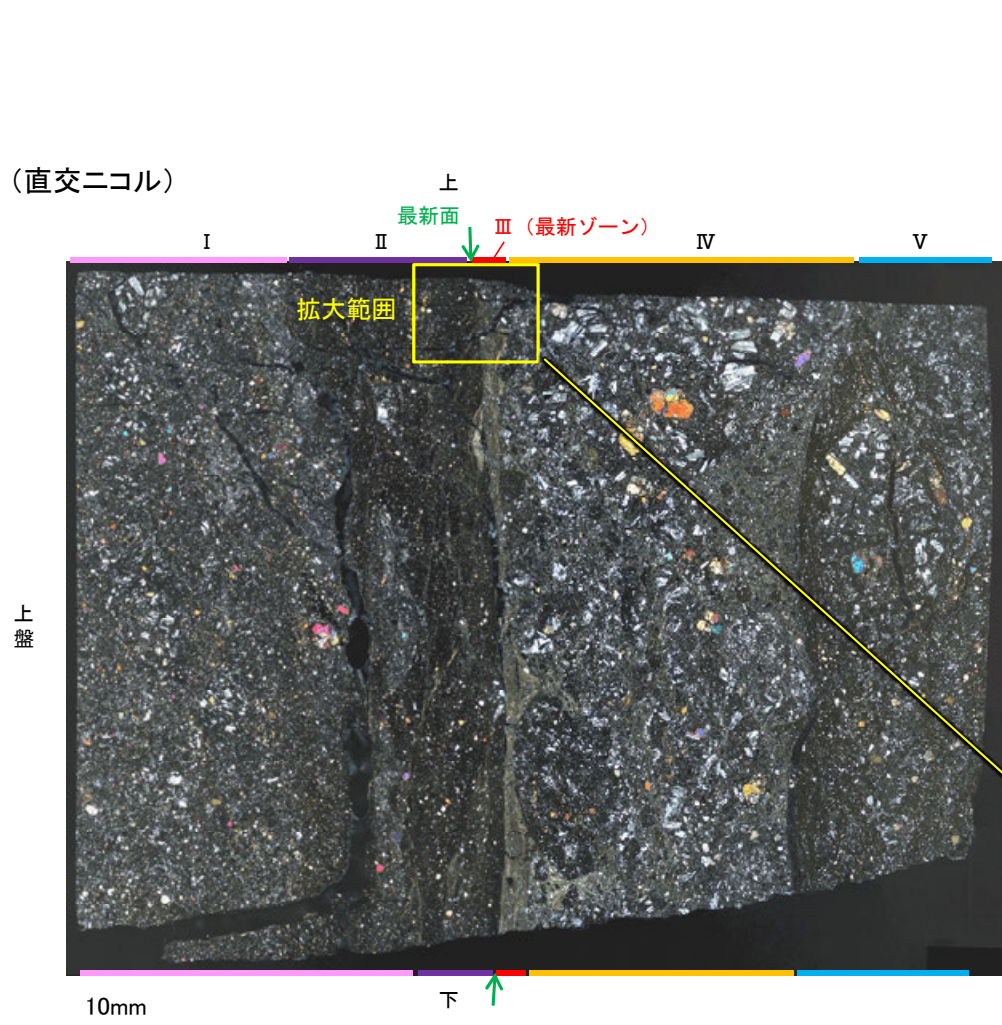
観察用薄片写真(E-8.60_126R)
