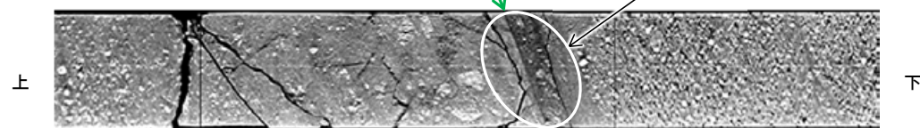
CT画像 (E-8.60孔)
