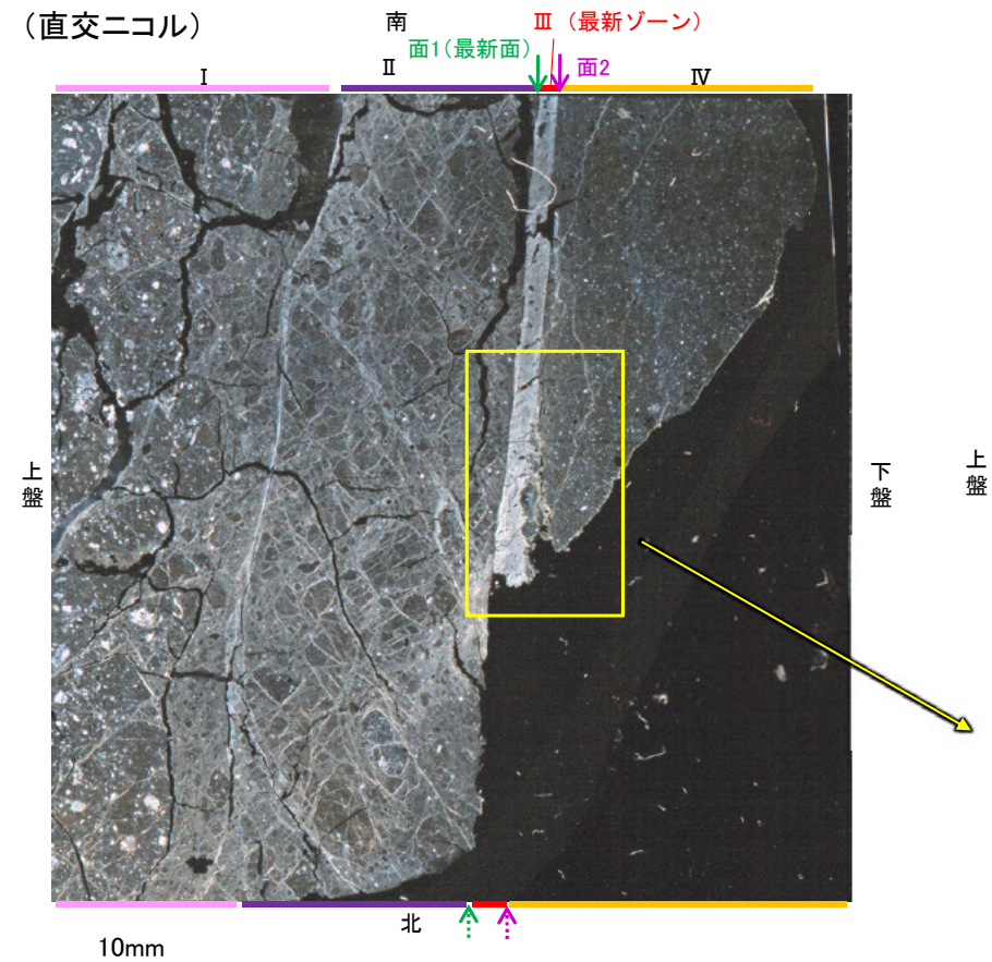
薄片写真(E-8.5-2_0R)
