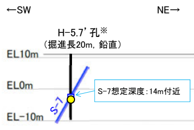
H-5.7'孔断面図 (断層直交方向, H:V=1:1)
