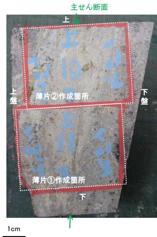
ブロック写真
