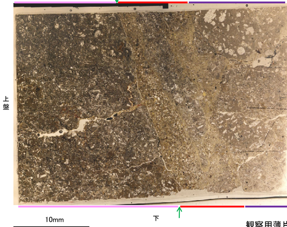
観察用薄片写真(H-5.4-1E_78R)
