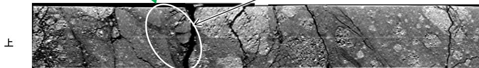
CT画像(H-5.4-1E孔)
