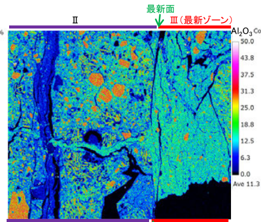
Al 2 O 3
