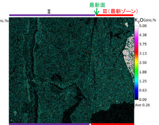
K 2 O
