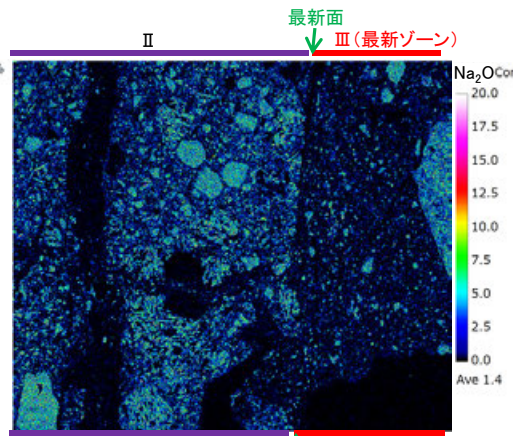
Na 2 O
