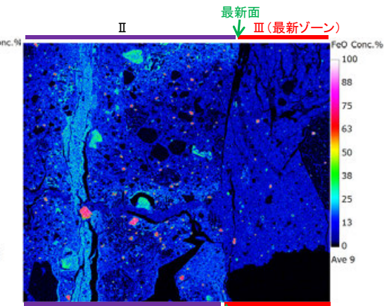
FeO
