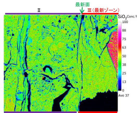
SiO 2
