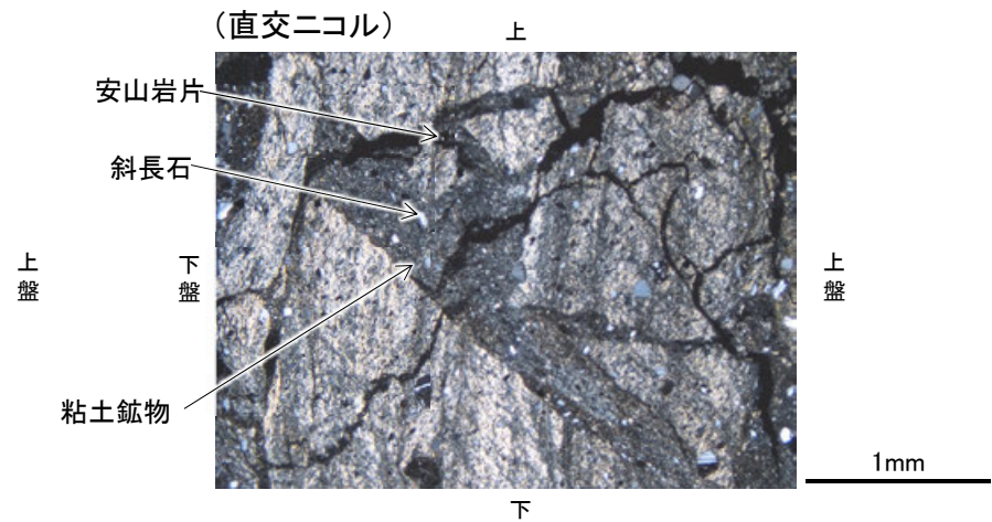
砕屑岩脈の構成物
