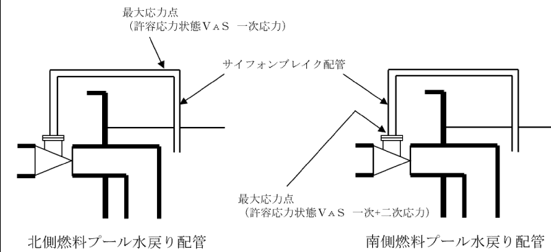
図6-1 最大応力点位置
