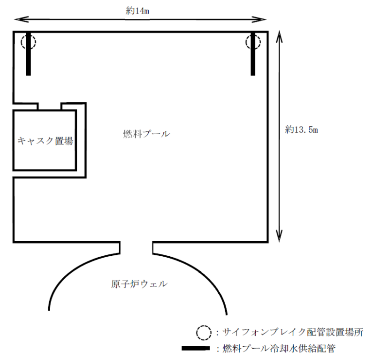
図 5-5 サイフォンブレイク配管の設置位置
