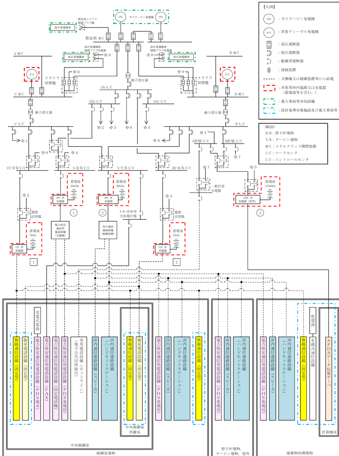
別図 通信連絡設備の電源概略構成図 (1/2)
