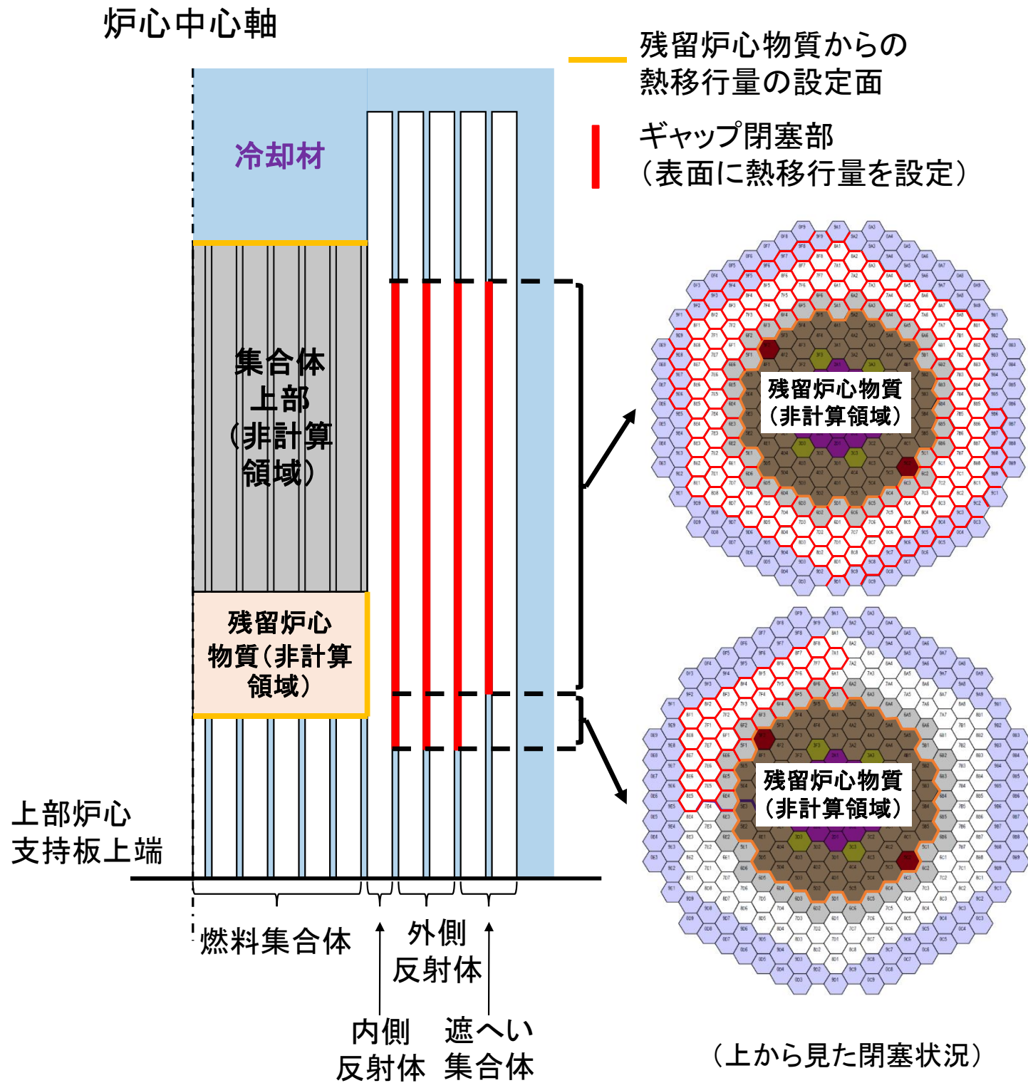
FLUENTにおけるギャップ閉塞部のモデル化概念図
