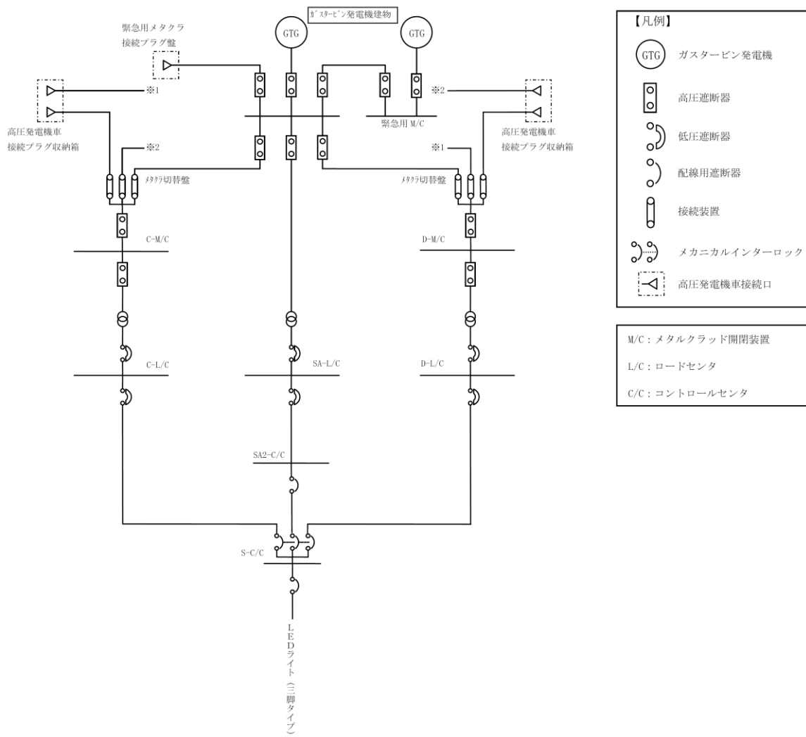
図 3-2 LED ライト（三脚タイプ）電源系統図
