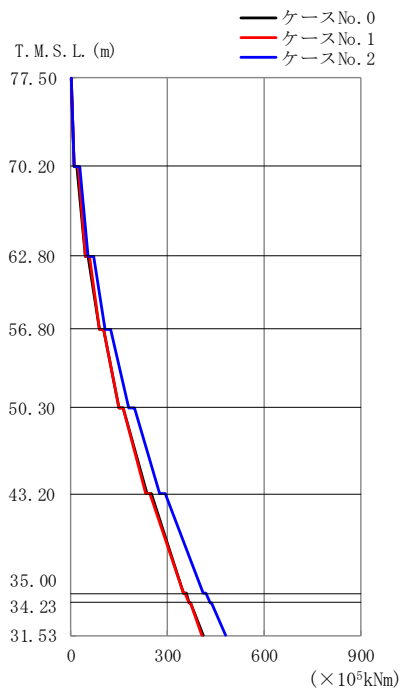
第4.2-23図 最大応答曲げモーメント (NS方向) (2/2)
