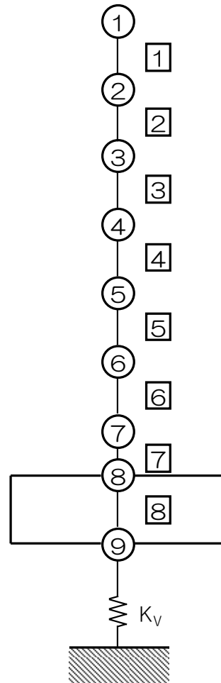
第 3. -2 図 地震応答解析モデル (鉛直方向)
