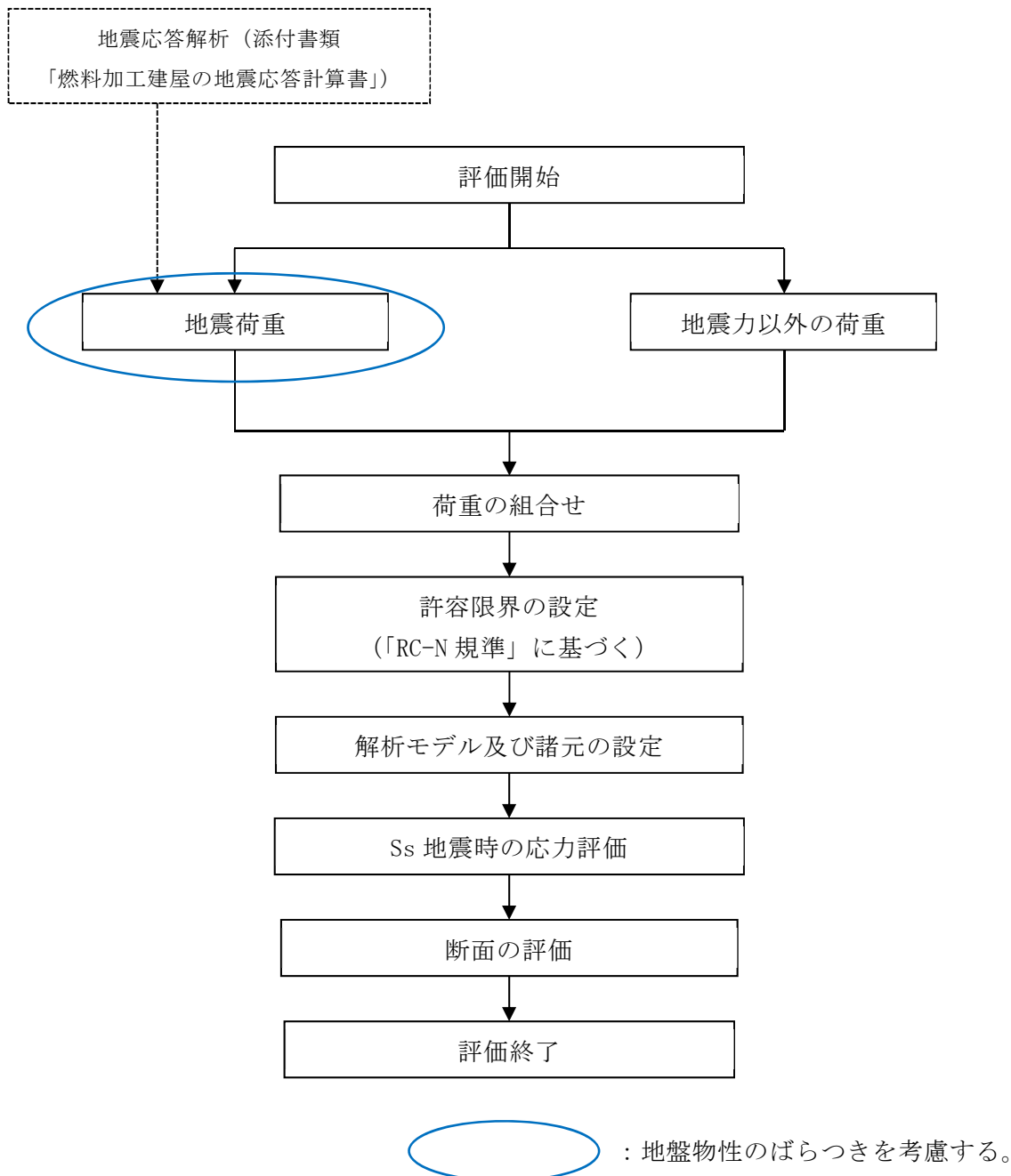
第 3.3-1 図 応力解析による評価フロー例（燃料加工建屋の基礎スラブ）
