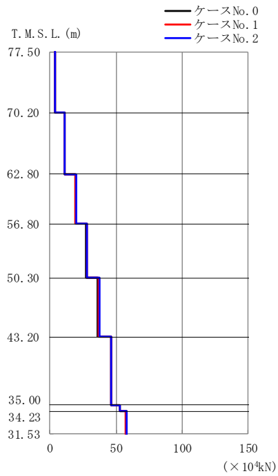
第 4.2-30 図 最大応答軸力 (鉛直方向) (1/2)
