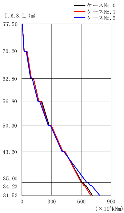
第4.2-4図 最大応答曲げモーメント (NS方向) (2/2)
