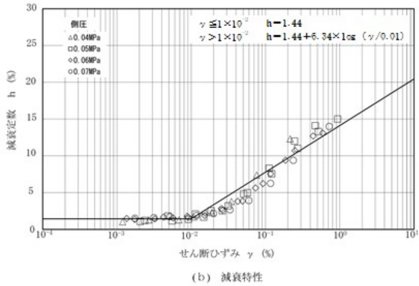
第 2. -4 図 造成盛土のひずみ依存特性 (「耐震建物 08 地震応答解析における地盤モデル及び物性値の設定について」の 別紙 1-1 第 2. 2. 2-1 図の再掲)
