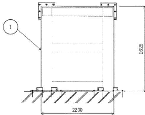
正面図
