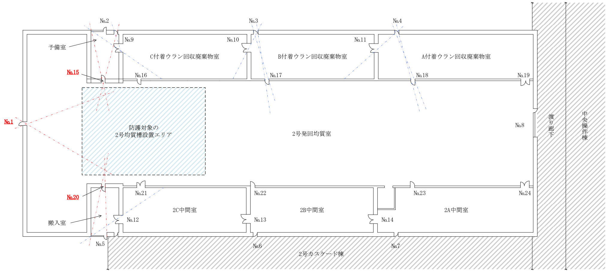
補足図-1 2号均質槽と開口部, 設計飛来物導線
