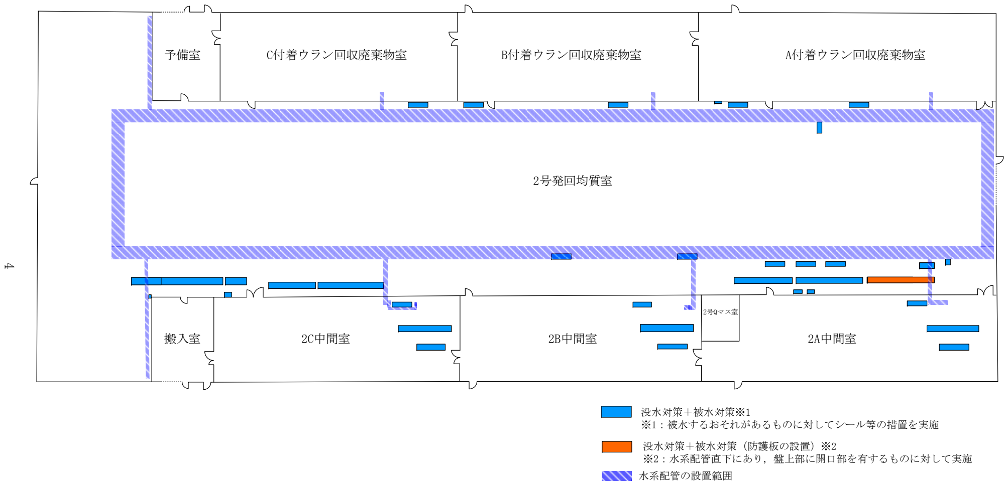
補足図4 盤と水系配管の配置概要図
