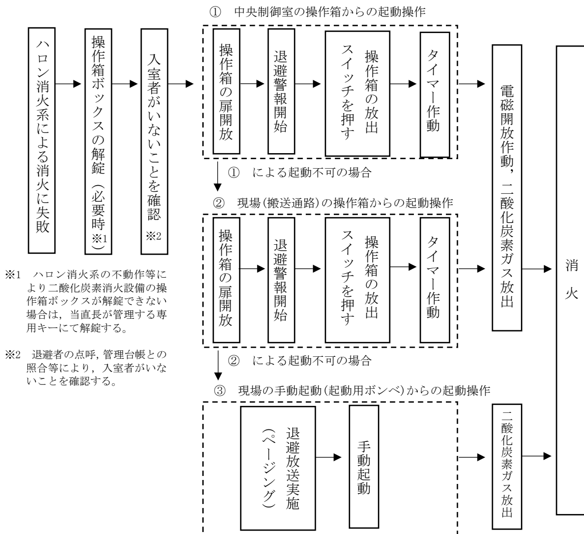
補足図 3 二酸化炭素消火系の作動の流れ
