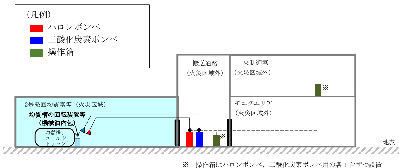
補足図1 遠隔消火設備の設計概要図
