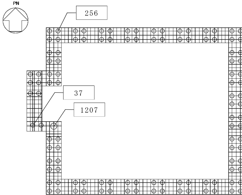
第 4-11 図 最大検定値発生位置（支持力及び引拔力）
