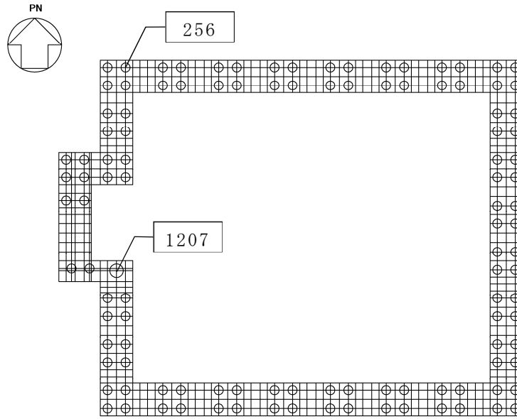
第 4-8 図 最大検定値発生位置（杭応力）
