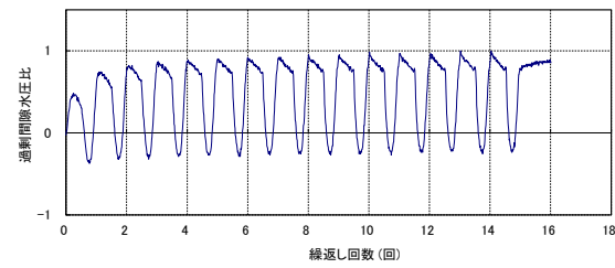
第 2-24 図 液状化強度試験結果 (KD-14_2-2 試料(供試体 No. 1))
