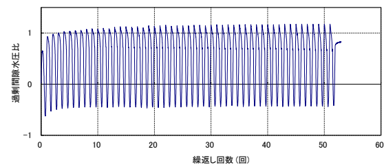
第 2-14 図 液状化強度試験結果 (KT-5_6 試料(供試体 No. 3))
