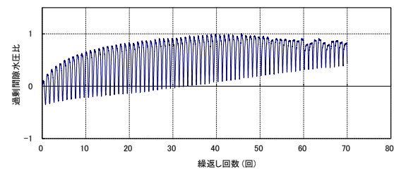
第 2-34 図 液状化強度試験結果 (KD-20_2-2 試料(供試体 No. 3))
