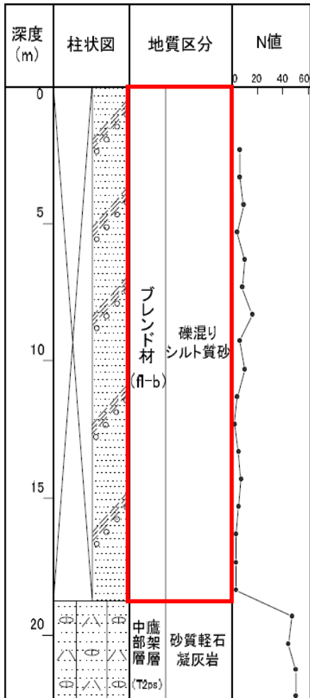
第1-5図 ボーリング柱状図・コア写真 (KD-20)
