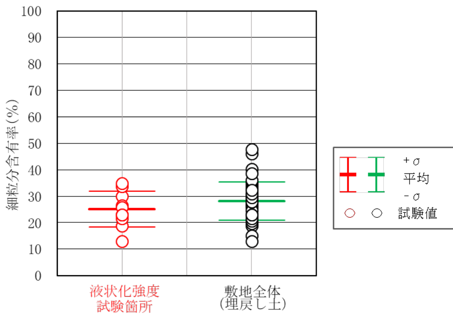
第 4-5 図 埋戻し土の細粒分含有率の比較
