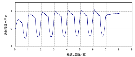
第 2-27 図 液状化強度試験結果 (KD-14_2-2 試料(供試体 No. 4))
