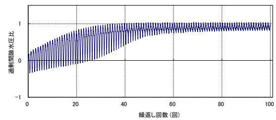
第 2-20 図 液状化強度試験結果 (KT-9_2-2-4 試料(供試体 No. 1))
