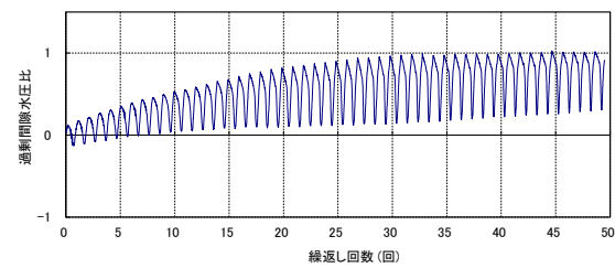
第 2-36 図 液状化強度試験結果 (KD-20_5-2 試料(供試体 No. 1))
