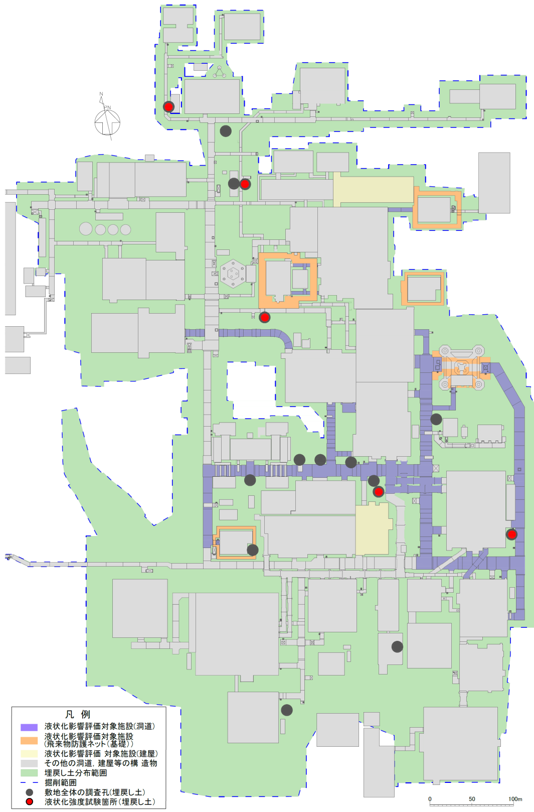
第 4-3 図 埋戻し土の液状化強度試験の試料採取位置
