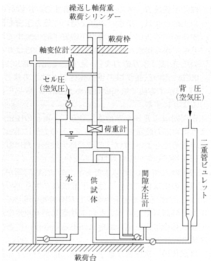
第 4-7 図 繰返し非排水三軸試験装置の概要
