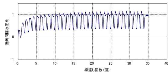
第 2-26 図 液状化強度試験結果 (KD-14_2-2 試料(供試体 No. 3))
