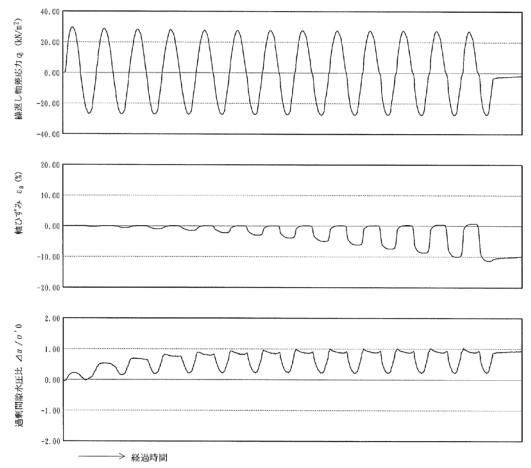
第 2-8 図 液状化強度試験結果 (KT-3_5-2 試料(供試体 No. 4))
