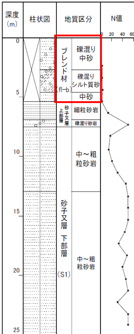
第1-3図 ボーリング柱状図・コア写真 (KT-9)
