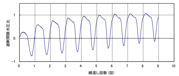
第 2-35 図 液状化強度試験結果 (KD-20_2-2 試料(供試体 No. 4))
