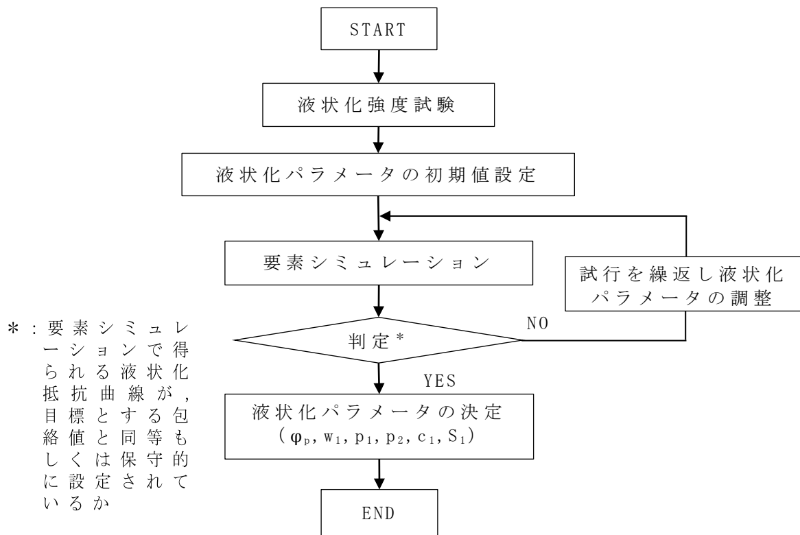
第 4-13 図 FLIP における液状化パラメータの設定フロー
