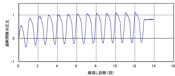
第 2-18 図 液状化強度試験結果 (KT-5_11 試料(供試体 No. 3))
