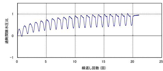
第 2-16 図 液状化強度試験結果 (KT-5_11 試料(供試体 No. 1))
