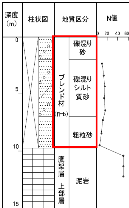
第 1-1 図 ボーリング柱状図・コア写真 (KT-3)
