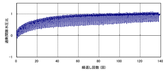
第 2-11 図 液状化強度試験結果 (KT-5_4 試料(供試体 No. 3))
