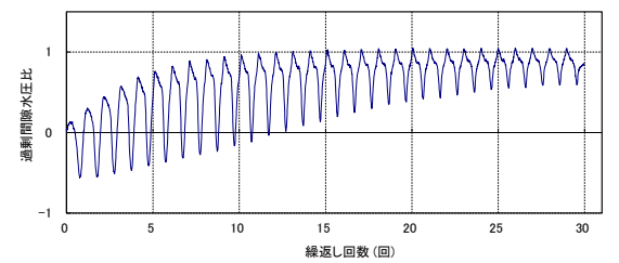
第 2-23 図 液状化強度試験結果 (KT-9_2-2-4 試料(供試体 No. 4))
