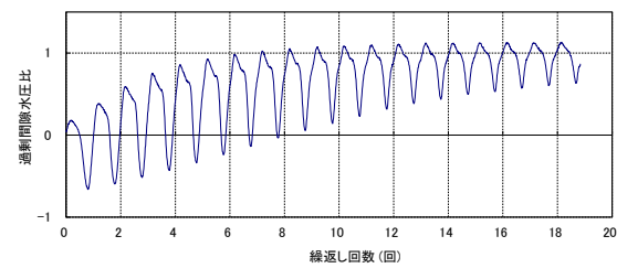
第 2-22 図 液状化強度試験結果 (KT-9_2-2-4 試料(供試体 No. 3))
