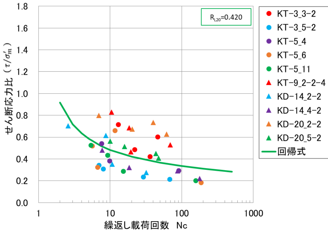
第 4-10 図 埋戻し土の液状化強度試験結果及び R_{L20}
