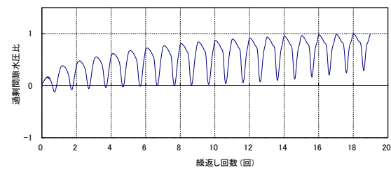
第 2-38 図 液状化強度試験結果 (KD-20_5-2 試料(供試体 No. 3))
