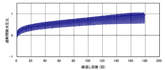
第 2-19 図 液状化強度試験結果 (KT-5_11 試料(供試体 No. 4))
