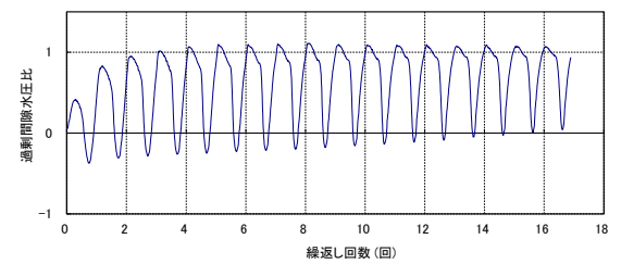
第 2-37 図 液状化強度試験結果 (KD-20_5-2 試料(供試体 No. 2))
