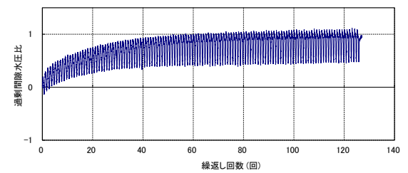
第 2-31 図 液状化強度試験結果 (KD-14_4-2 試料(供試体 No. 4))
