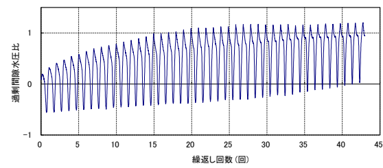
第 2-32 図 液状化強度試験結果 (KD-20_2-2 試料(供試体 No. 1))
