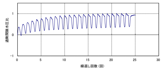
第 2-29 図 液状化強度試験結果 (KD-14_4-2 試料(供試体 No. 2))
