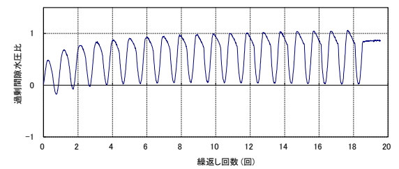
第 2-17 図 液状化強度試験結果 (KT-5_11 試料(供試体 No. 2))
