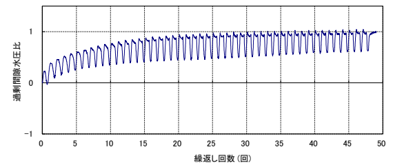
第 2-25 図 液状化強度試験結果 (KD-14_2-2 試料(供試体 No. 2))
