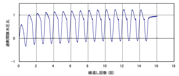
第 2-15 図 液状化強度試験結果 (KT-5_6 試料(供試体 No. 4))
