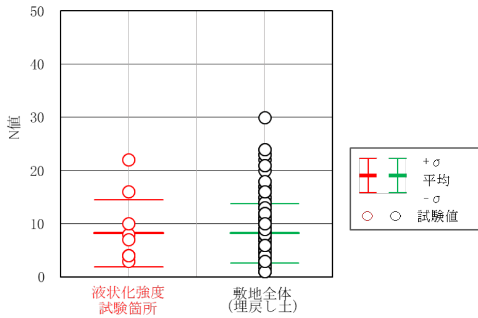
第 4-6 図 埋戻し土の N 値の比較
