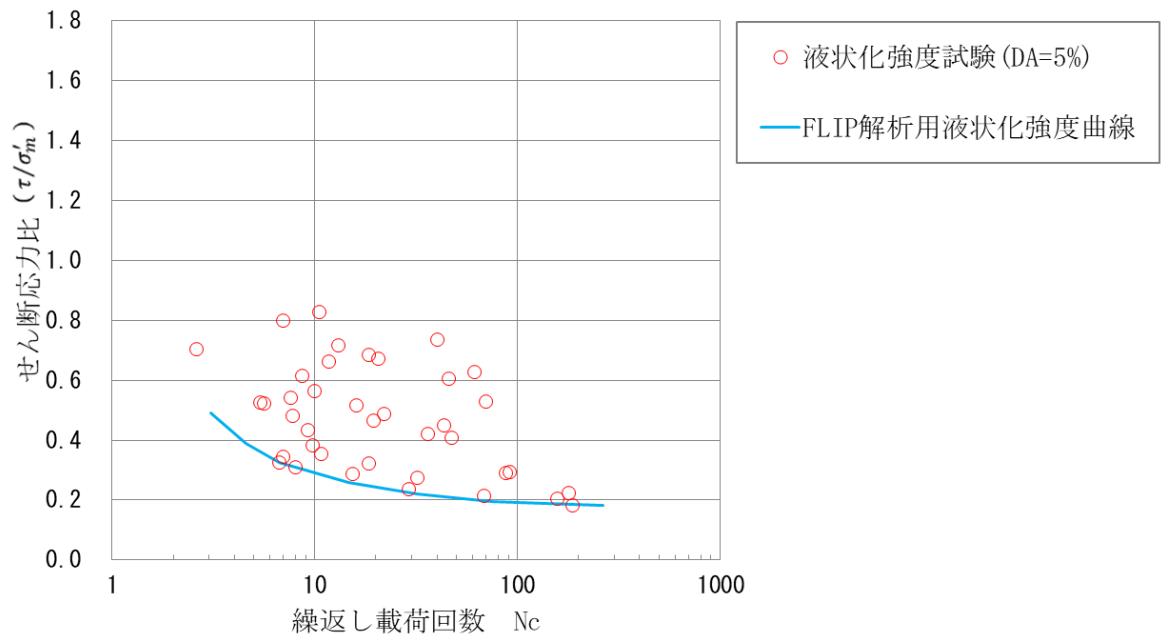
第 4-14 図 液状化強度試験結果と液状化強度特性の設定（埋戻し土）
