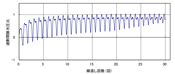
第 2-21 図 液状化強度試験結果 (KT-9_2-2-4 試料(供試体 No. 2))
