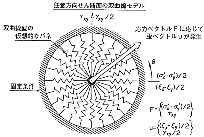
第 4-11 図 マルチスプリング・モデルの概念図 (引用：港湾技研資料 N0.869 「液状化による構造物被害予測プログラム FLIP において必要な各種パラメタの簡易設定法」, 1997.4)
