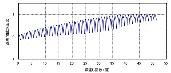
第 2-39 図 液状化強度試験結果 (KD-20_5-2 試料(供試体 No. 4))
