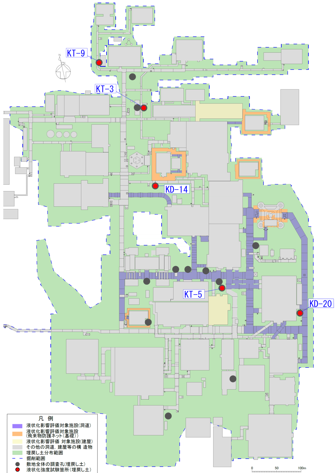
第 4-8 図 埋戻し土の液状化強度試験の試料採取位置とボーリング孔名
