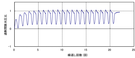
第 2-12 図 液状化強度試験結果 (KT-5_6 試料(供試体 No. 1))
