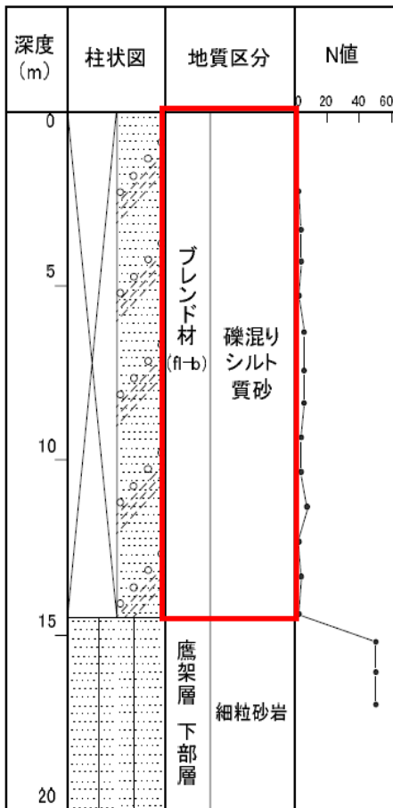
第 1-2 図 ボーリング柱状図・コア写真 (KT-5)
