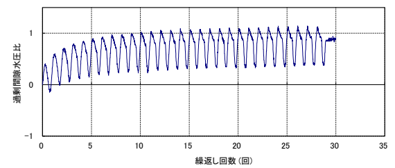
第 2-10 図 液状化強度試験結果 (KT-5_4 試料(供試体 No. 2))
