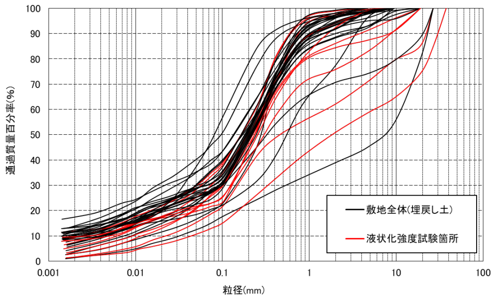
第 4-4 図 埋戻し土の粒度分布の比較
