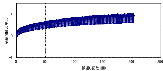
第 2-30 図 液状化強度試験結果 (KD-14_4-2 試料(供試体 No. 3))
