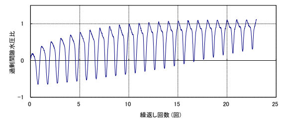
第 2-33 図 液状化強度試験結果 (KD-20_2-2 試料(供試体 No. 2))
