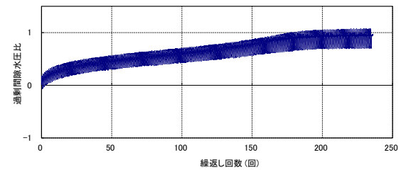
第 2-13 図 液状化強度試験結果 (KT-5_6 試料(供試体 No. 2))
