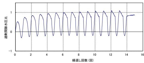
第 2-9 図 液状化強度試験結果 (KT-5_4 試料(供試体 No. 1))
