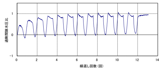
第 2-28 図 液状化強度試験結果 (KD-14_4-2 試料(供試体 No. 1))
