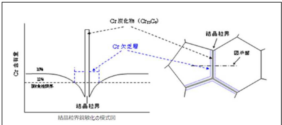
粒界腐食の模式図
