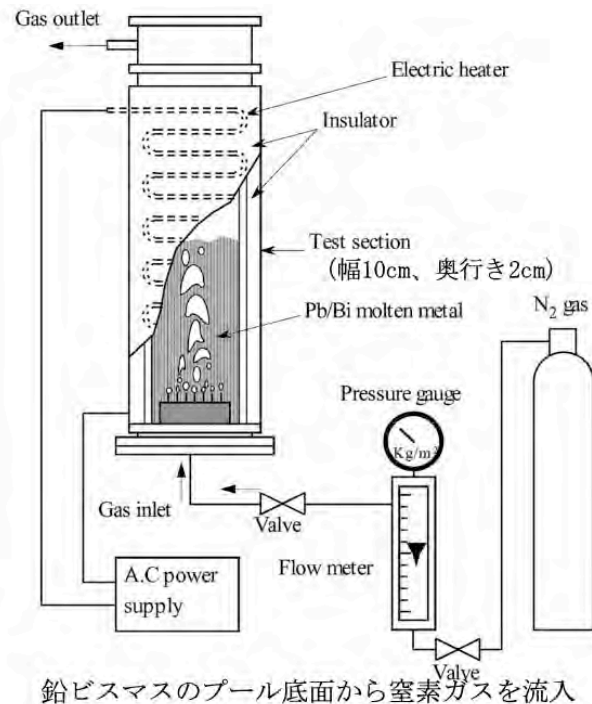
第 4.16 図 鉛ビスマス二相流動試験装置の概略図
