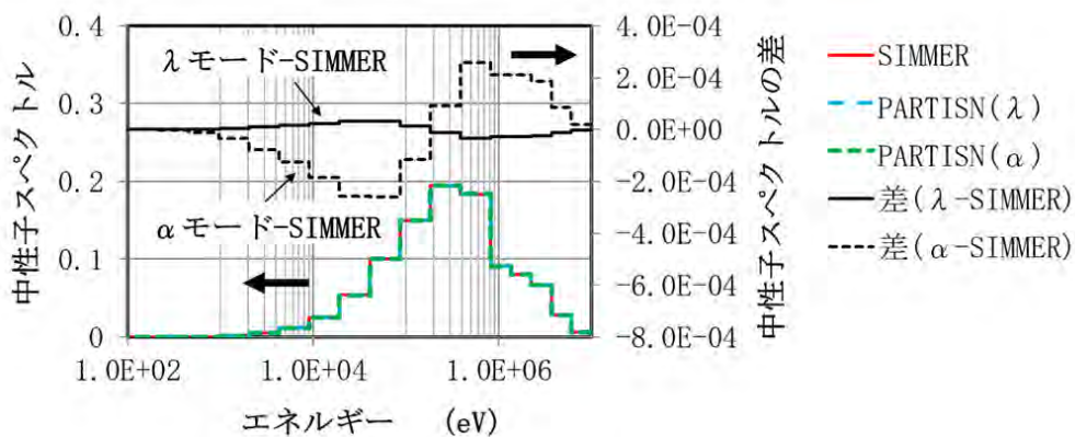
第 2.4 図 中性子スペクトルの比較
