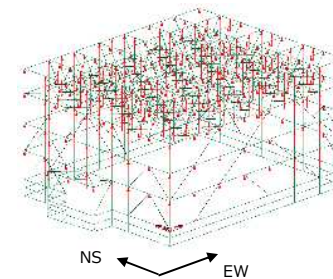
c. 地震荷重 (Ss) UD方向
