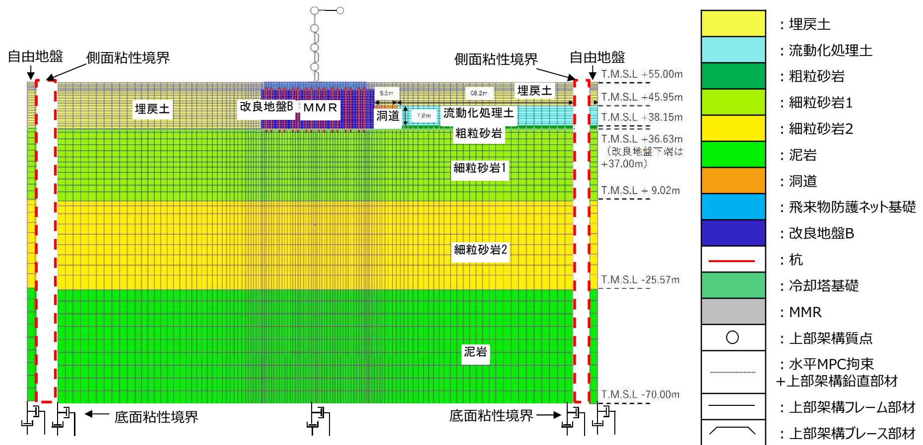
断面②-NS
