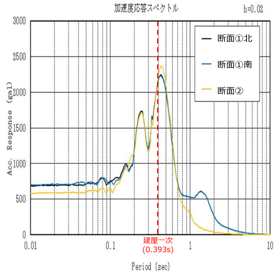
Ss-C1 (NS方向) - \sigma
