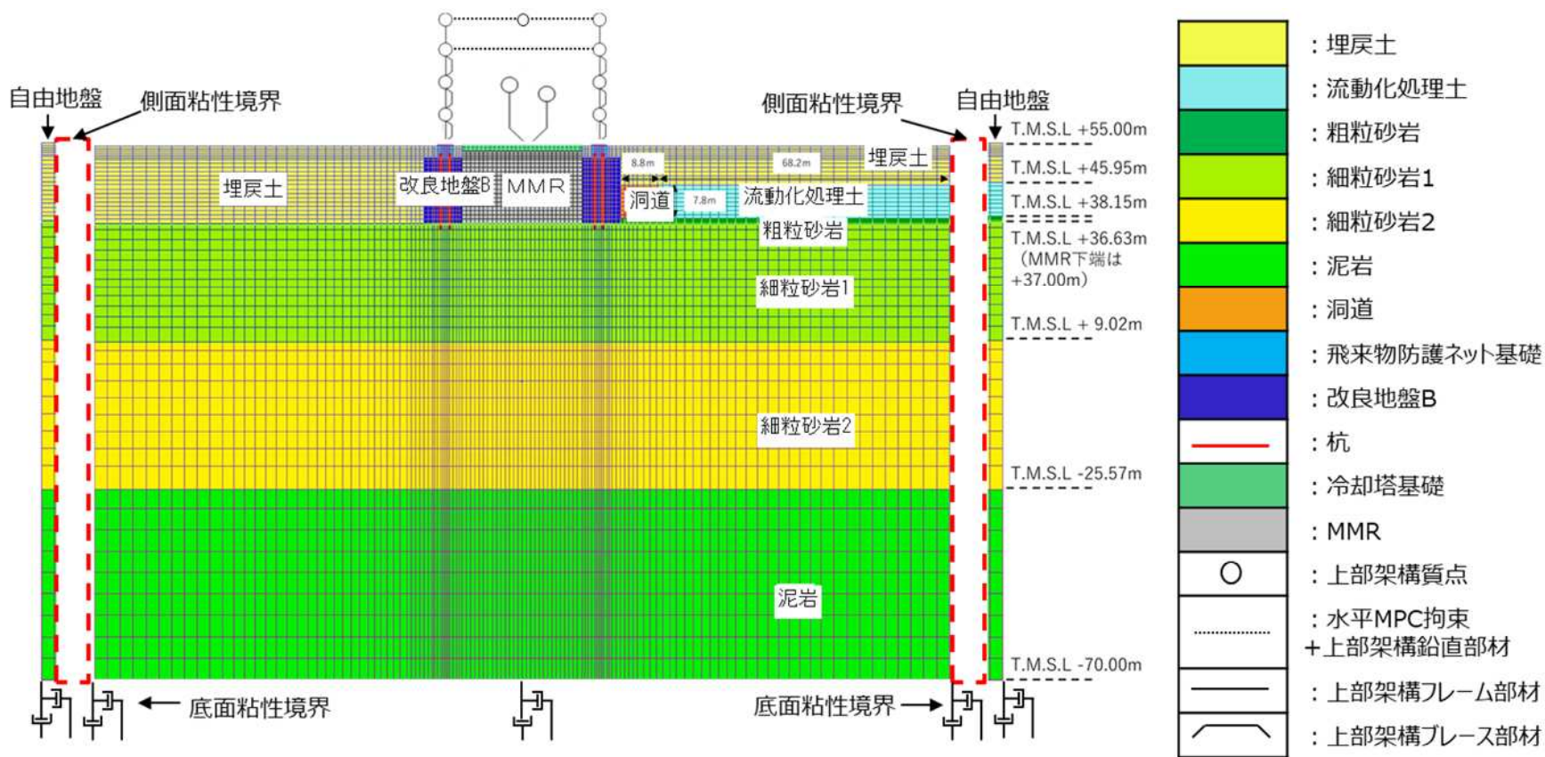
断面①-NS
