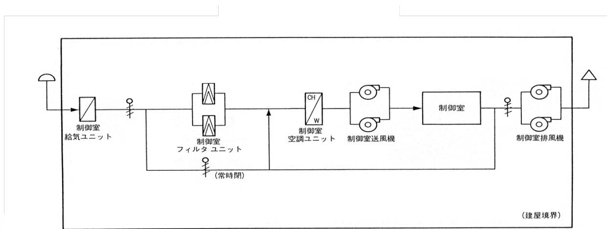
第1図 使用済燃料受入れ・貯蔵建屋制御室換気設備系統概要図
