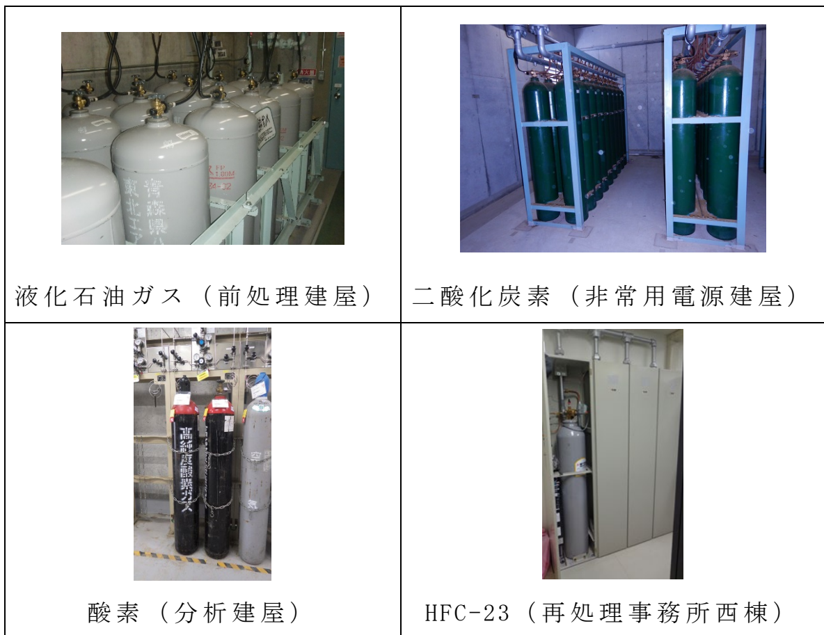
第2図 再処理施設における高圧ガス容器の保管状況
