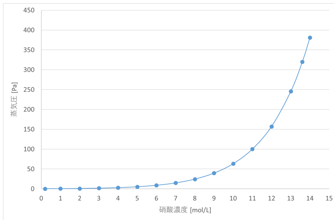
第6図 温度30°Cにおける硝酸濃度の違いによる蒸気圧の変化
