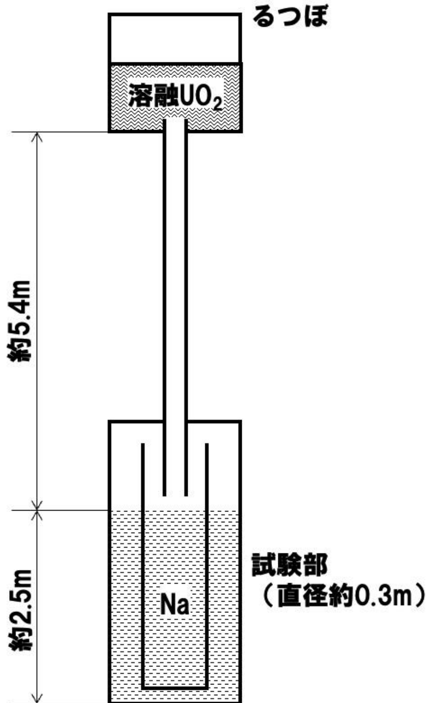
FARO-TERMOS試験装置の概念図
