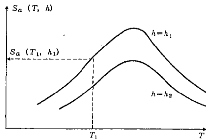
図 6.5.1-2 床応答スペクトル
