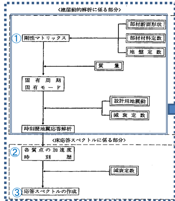
図 6.5.1-1 解析フロー図
