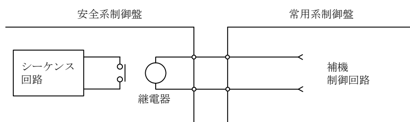
信号伝送における分離概念図
