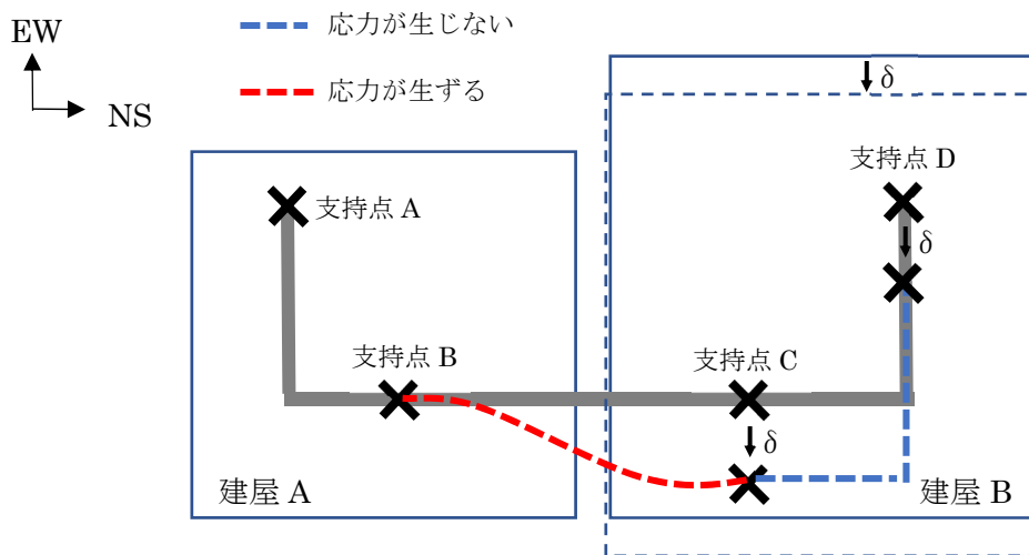
第 3.4.2.3-1 図 EW 方向の相対変位に対する配管挙動イメージ
