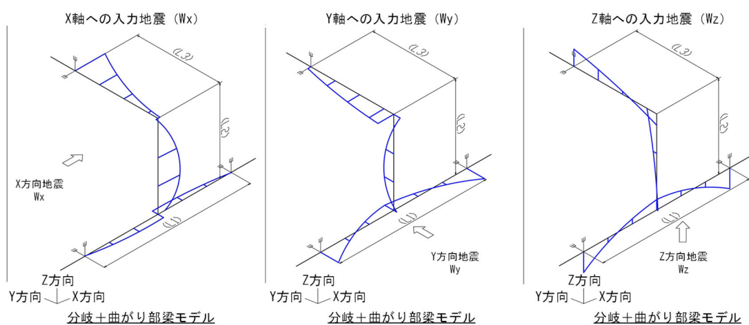
第3.4.2.2-13図 配管（分岐+曲がり部）モデル
