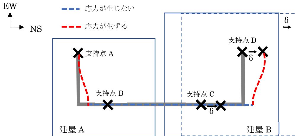
第3.4.2.3-2図 NS方向相対変位に対する配管挙動イメージ
