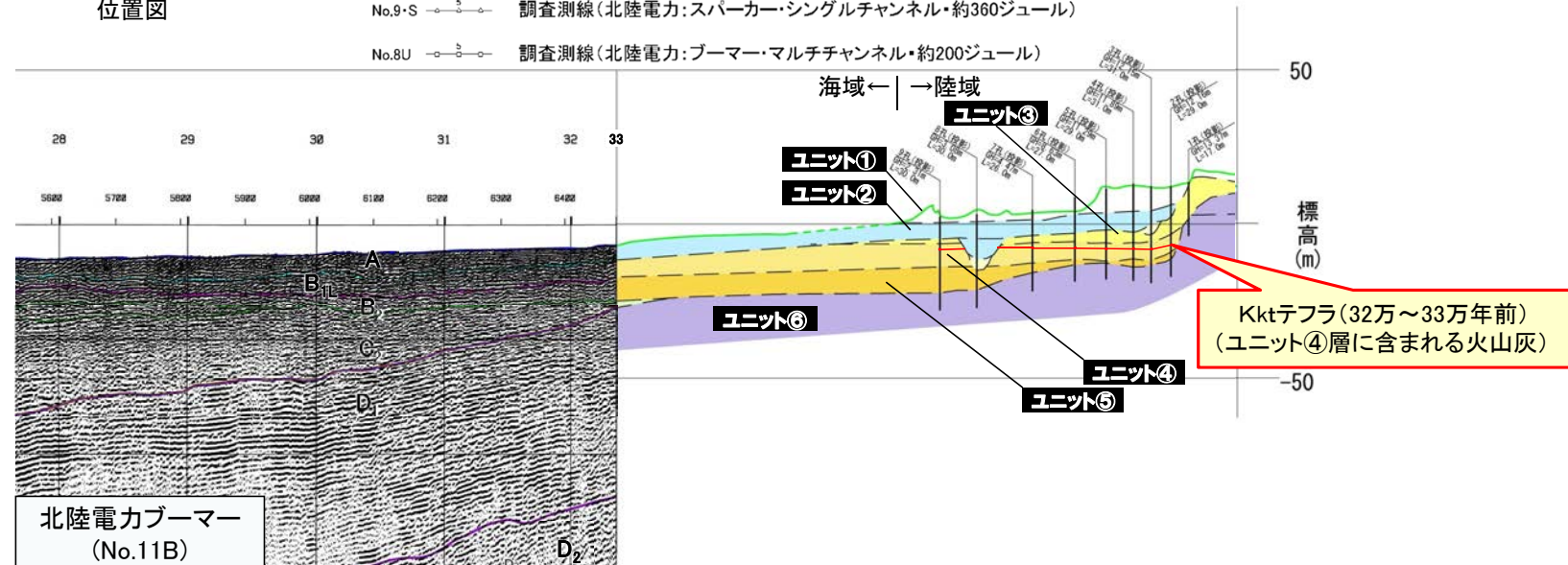
海域と陸域の地質層序
