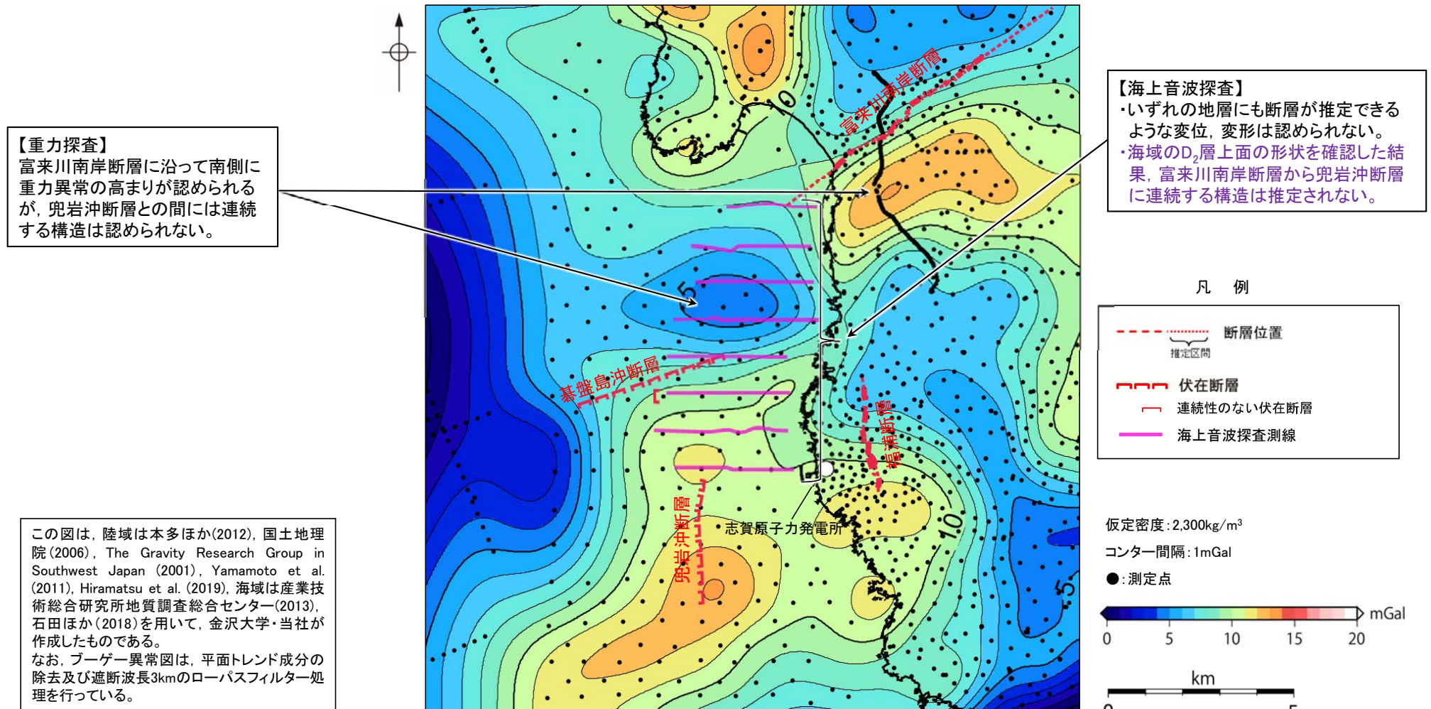
ブーゲー異常図
