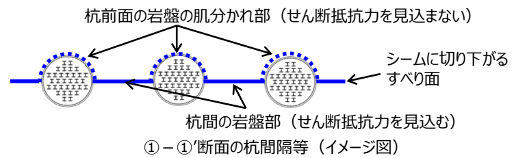
①-①'断面の杭間隔等 (イメージ図)
