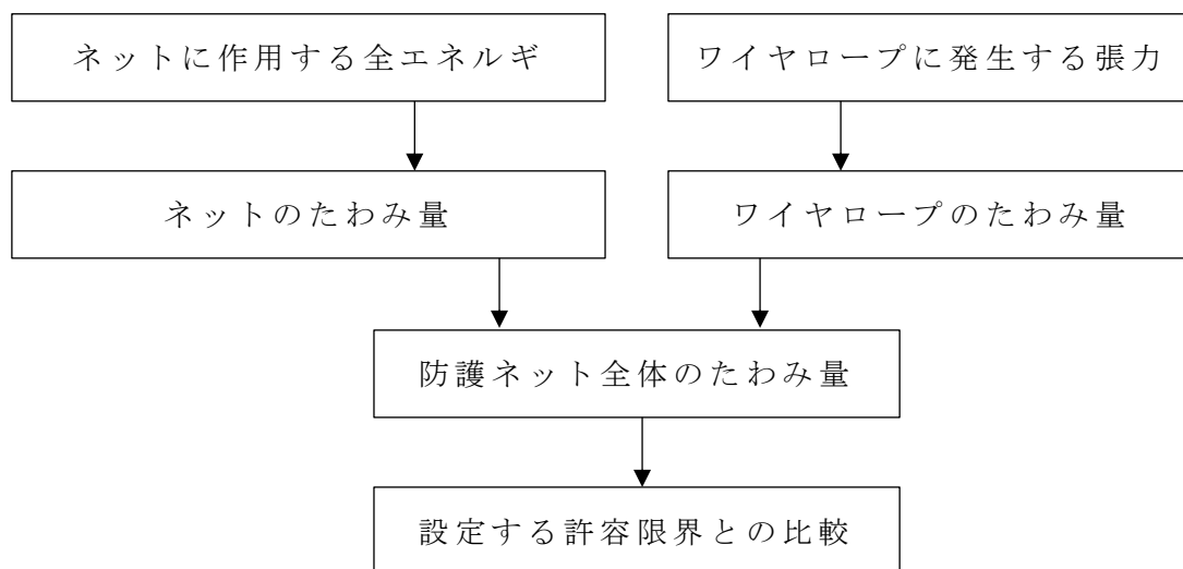
第3-2図 たわみ評価の評価フロー
