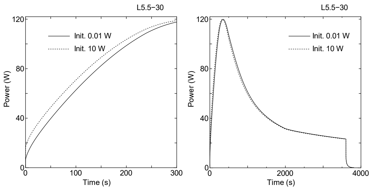
図1 L5.5P-30 炉心 初期出力を変化させた時の出力変化 (実線 : 0.01W、点線 10W) (両図は横軸のスケールの違い)
