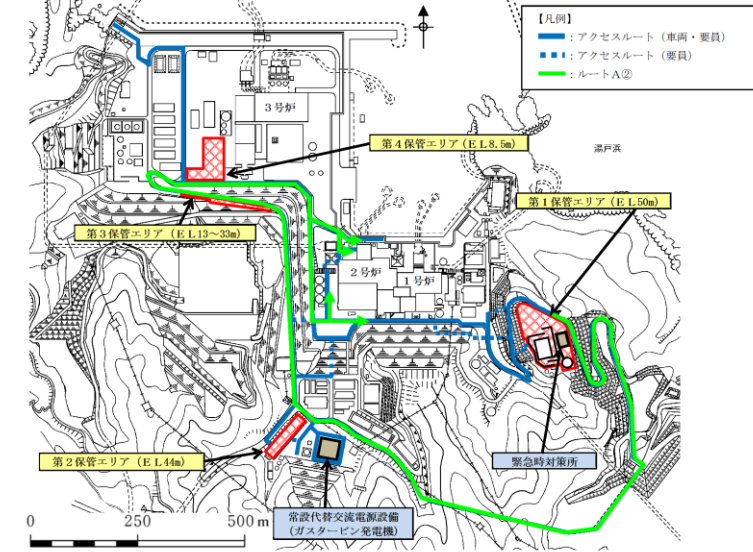
第2-4図 保管場所からのアクセスルート概要 (1 / 4)
