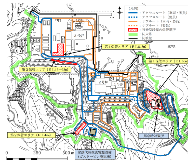
第 2-3 図 屋外アクセスルート図
