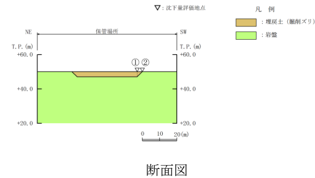
第3-12 図 第1保管エリアの傾斜評価地点
