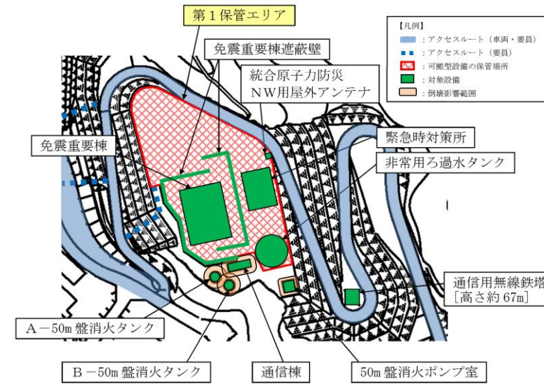
第3-2図(1) 第1保管エリア
