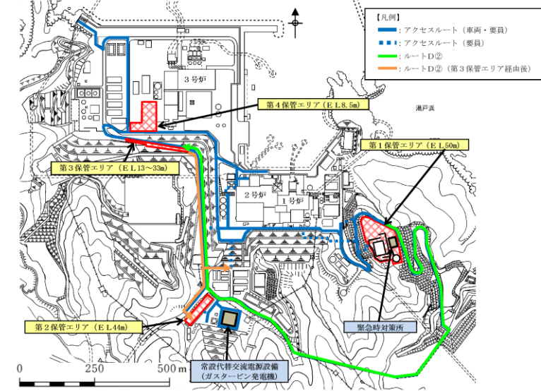
第2-4図 保管場所からのアクセスルート概要 (4 / 4)
