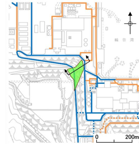
第 4.3-1 図 33m 盤盛土斜面の断面位置図
