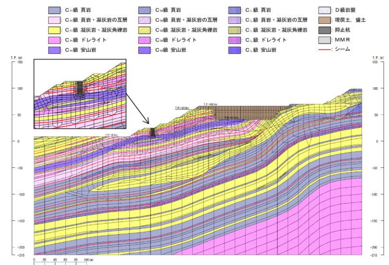
第 7. 4. 3-3(2) 図 ①-①' 断面 解析用要素分割図
