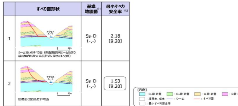
第 6.5-3 図 グループC (岩盤斜面, 法尻標高 T.P. +33~50m) のすべり安定性評価結果
