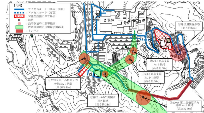
第4図 鉄塔倒壊によるアクセサルトへの影響想定 (66kV 鹿島支線, 220kV 第二島根原子力幹線, 通信用無線鉄塔)
