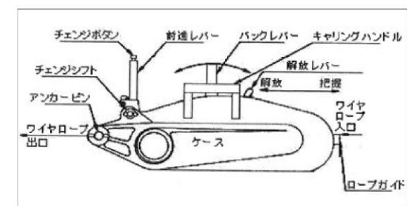
手動ウインチ構造図
