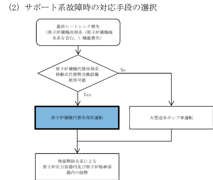
第 1.5-41 図 重大事故等時の対応手段選択フローチャート
