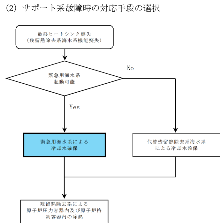
第 1.5-26 図 重大事故等時の対応手段選択フローチャート
