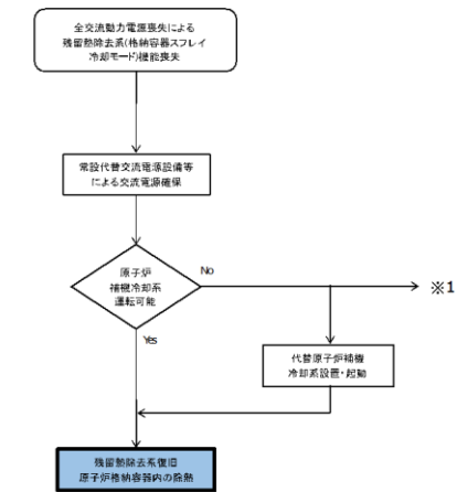
第 1.6.26 図 重大事故等発生時の対応手段選択フローチャート
