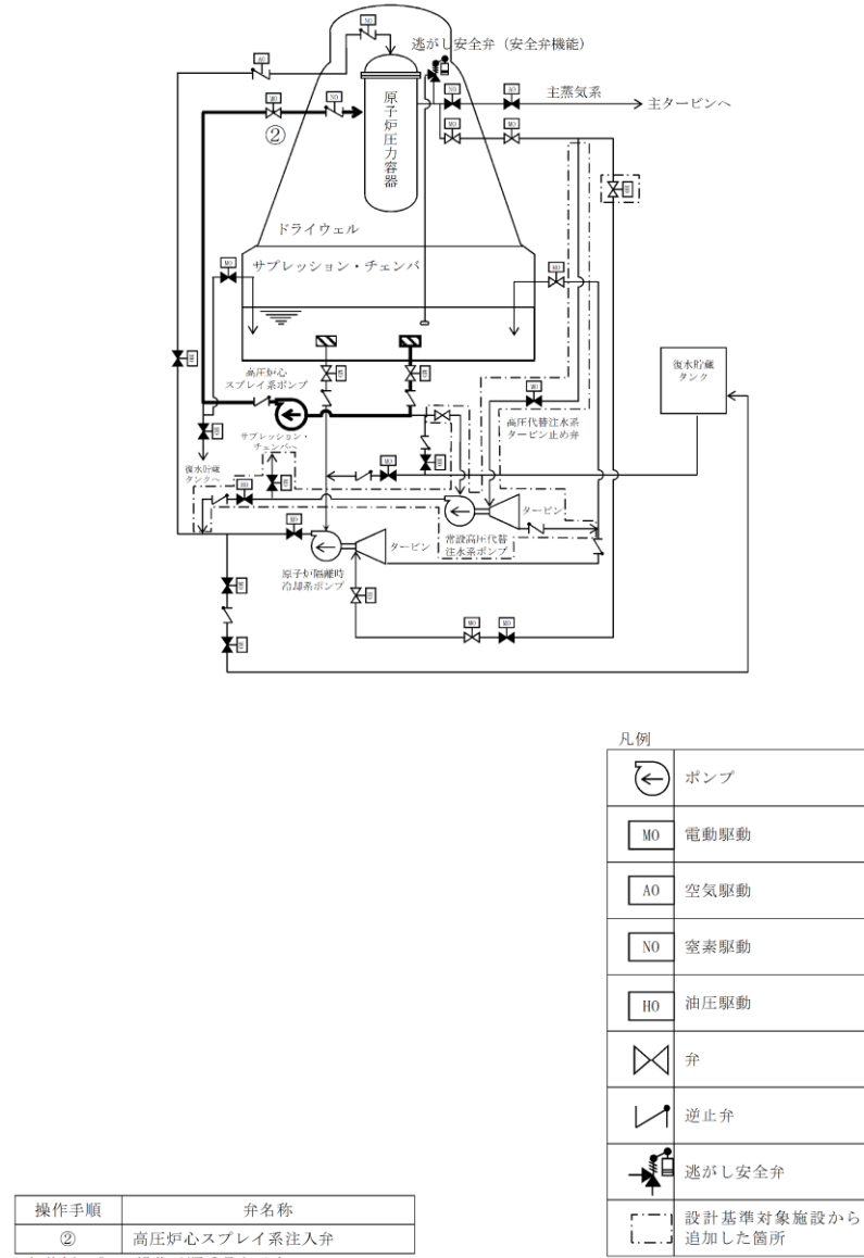
第 1.2-17 図 高圧炉心スプレィ系による原子炉圧力容器への注水 概要図
