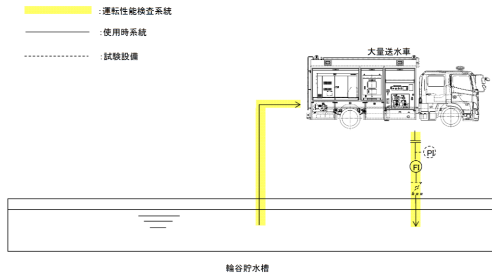
図 3 運転性能検査系統図 (大量送水車)
