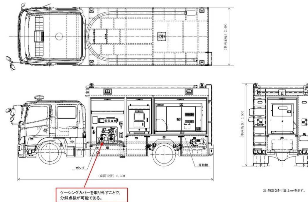
図 4 構造図 (大量送水車)
