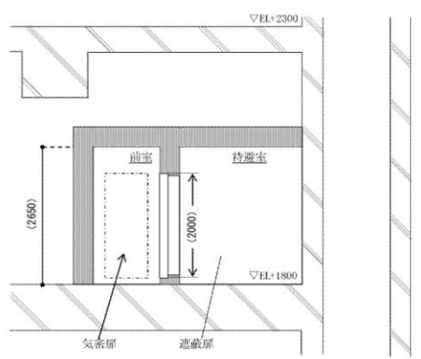
(A-A断面図)
