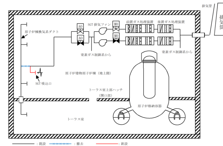
図1 SGT系統概要図
