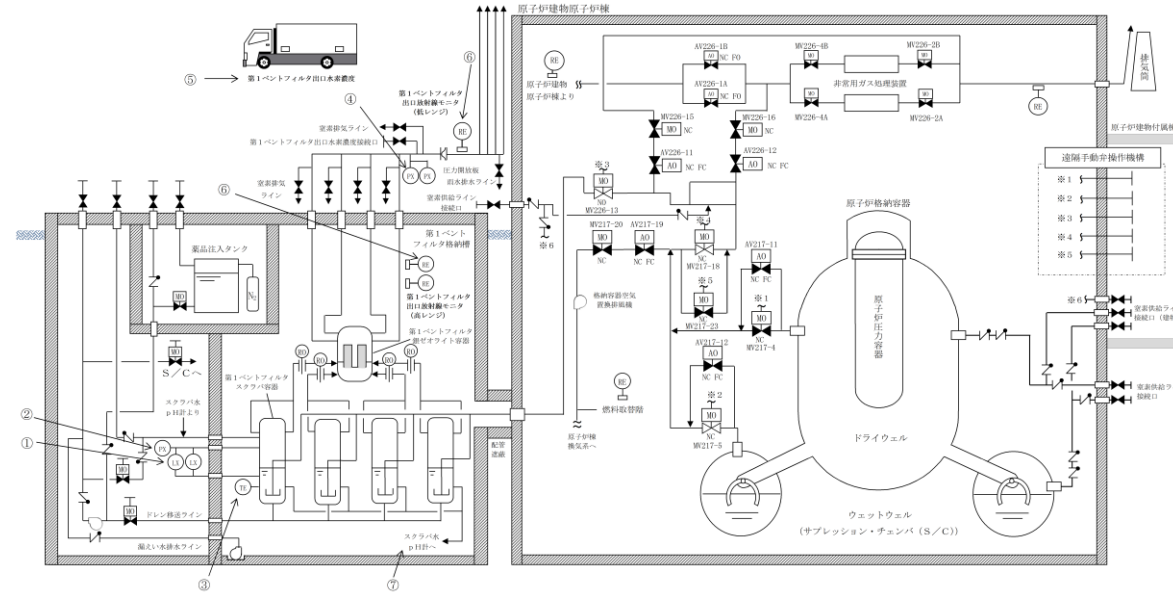
図1 格納容器フィルタバント系 計測制御系統図
