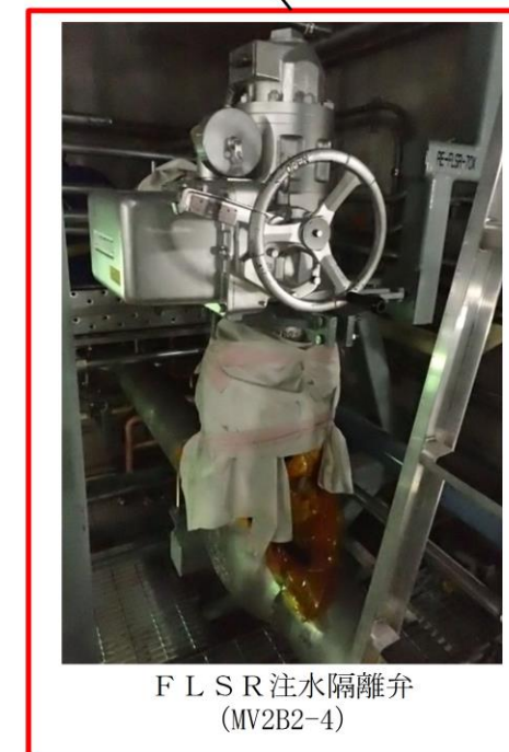
原子炉建物 1階 【EL.15300】
