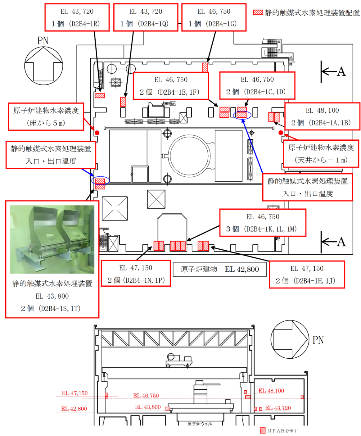
図1 機器配置図 (原子炉建物4階)
