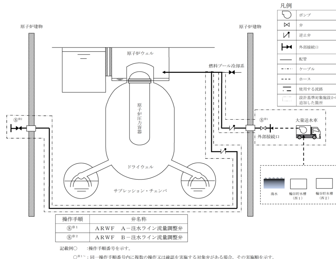
図1 原子炉ウェル代替注水系 概略図
