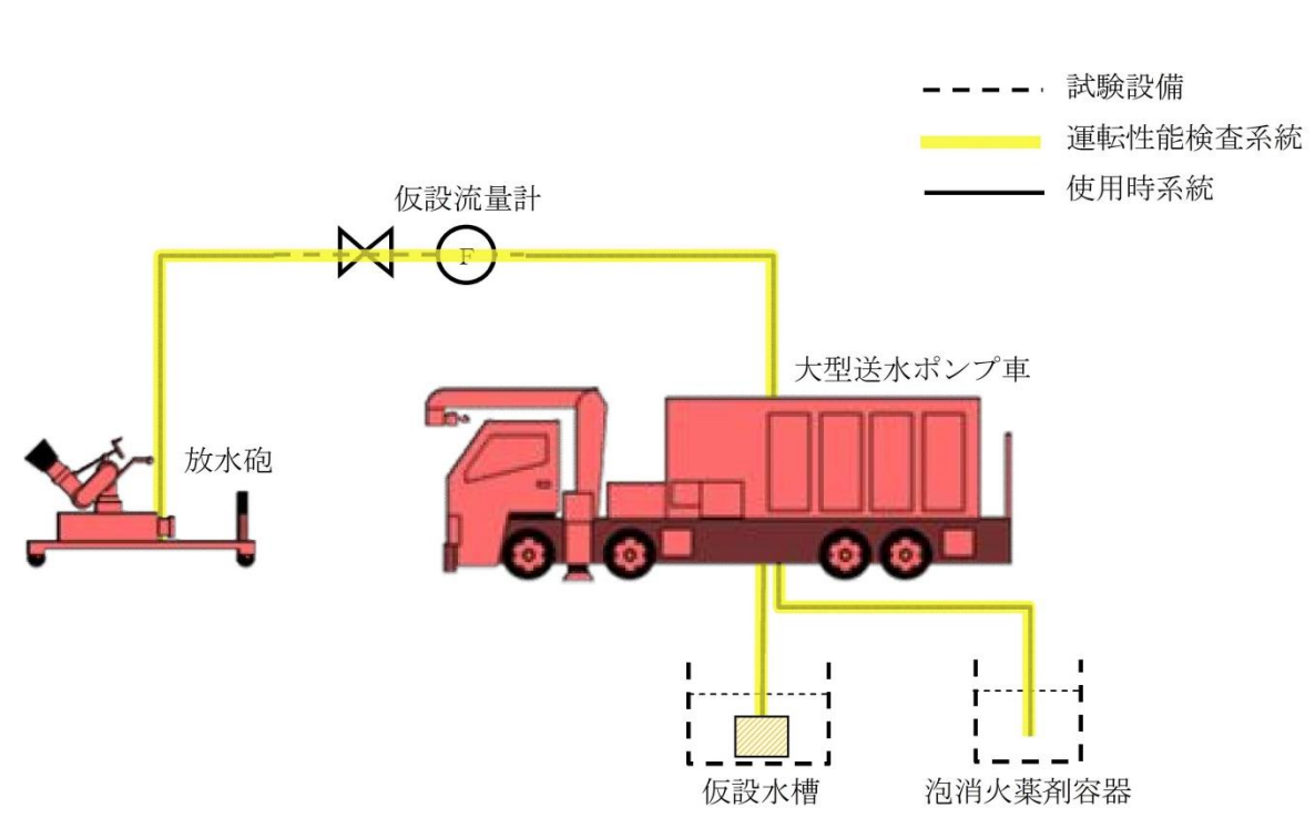
図 4-1 大型送水ポンプ車, 放水砲, 泡消火薬剤容器 試験系統図
