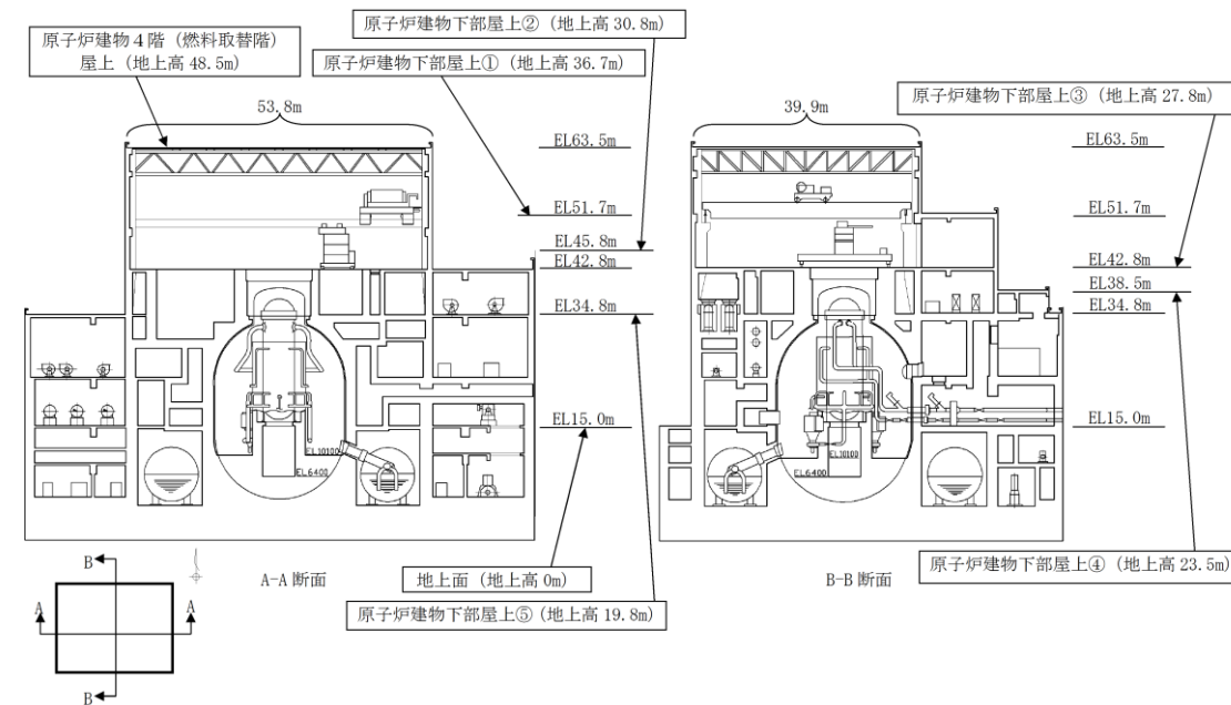
図 5-4 原子炉建物断面図
