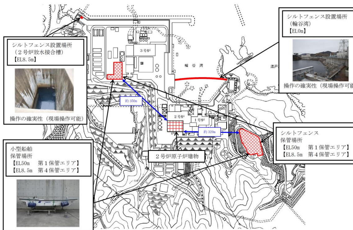
図 2-3 シルトフェンス, 小型船舶配置図
