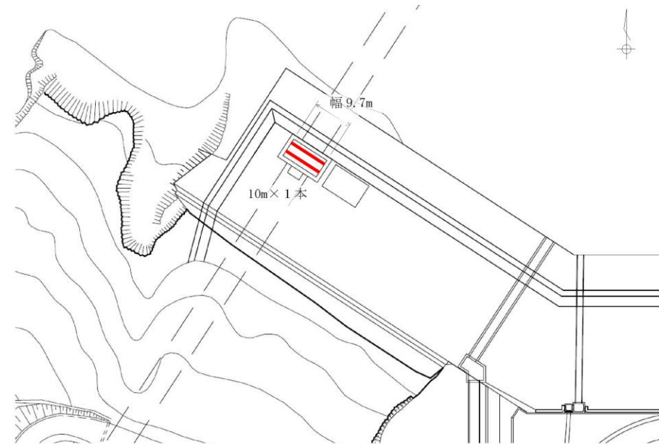
図 5-17 2号炉放水接合槽の外形図
