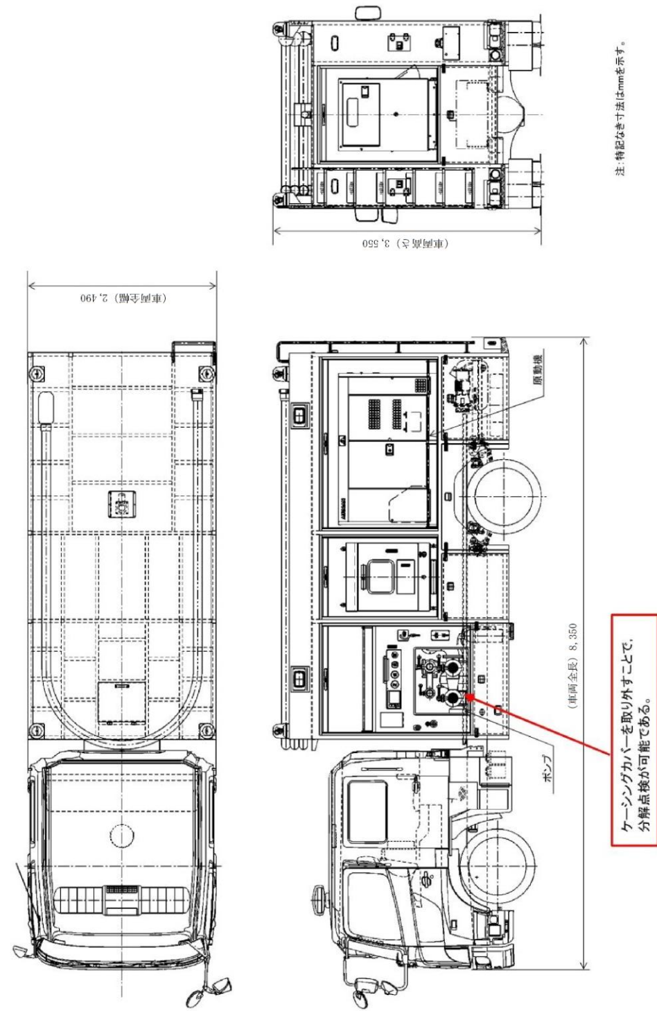
図2 大量送水車構造図
