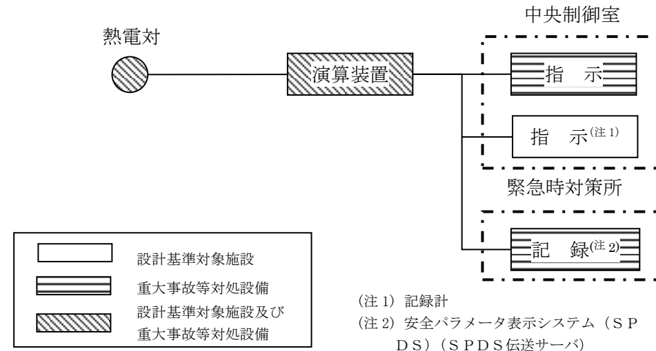
図2 燃料プール水位・温度 (SA) の概略構成図 (2)
