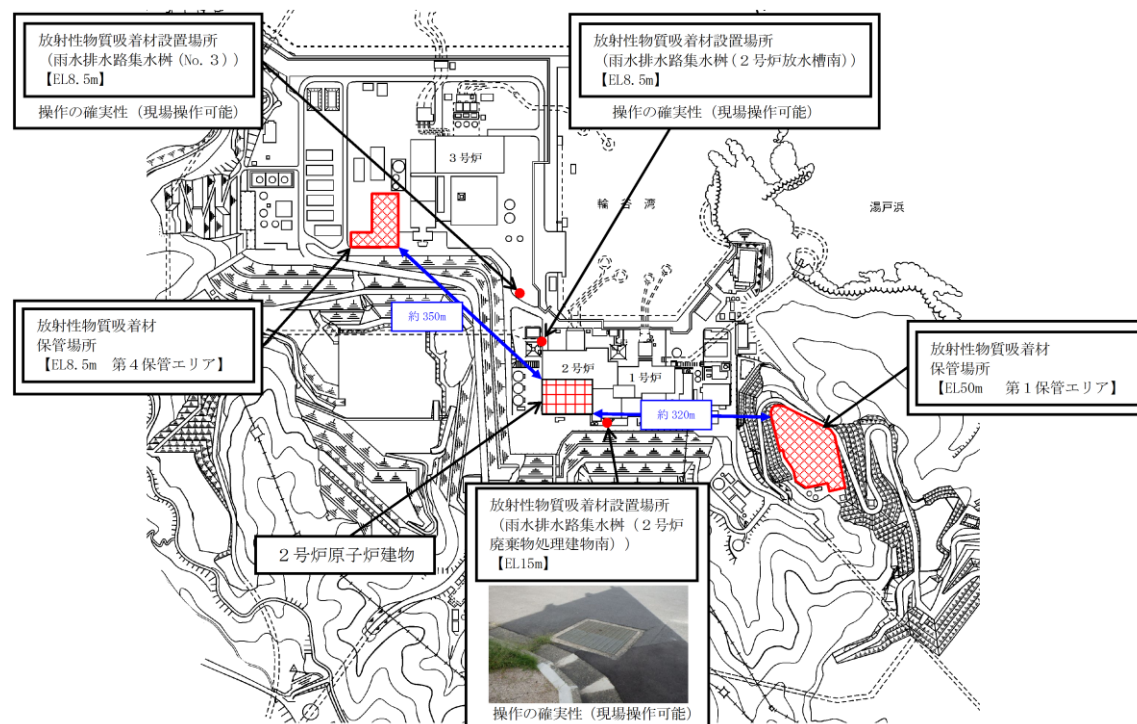
図 2-2 放射性物質吸着材配置図
