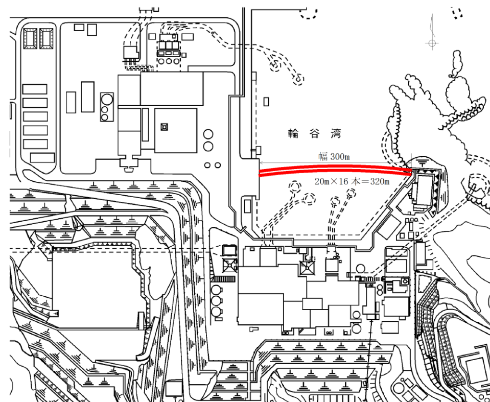
図 5-18 輪谷湾の外形図
