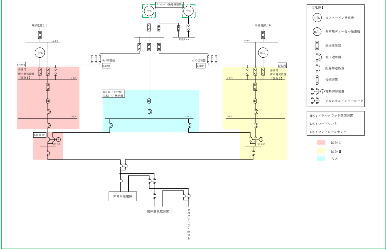
第 1.1-2 図 モニタリング・ポストの電源構成概略図等 (1 / 2)
