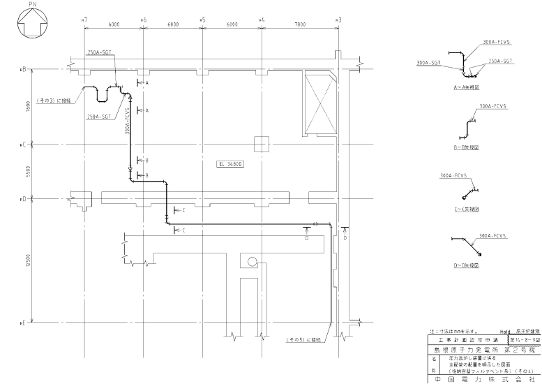
図 2.7.3-2 主配管の配置を明示した図面 (その 1)
