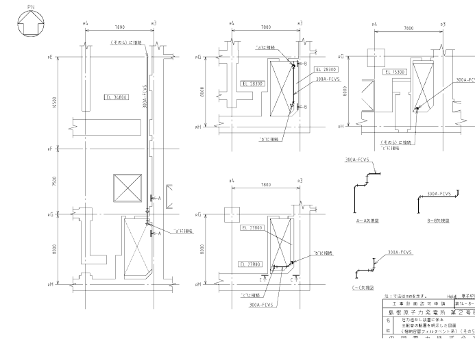
図 2.7.3-3 主配管の配置を明示した図面 (その 2)
