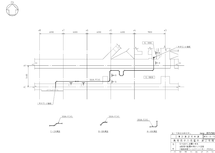
図 2.7.3-3 主配管の配置を明示した図面 (その 2)
