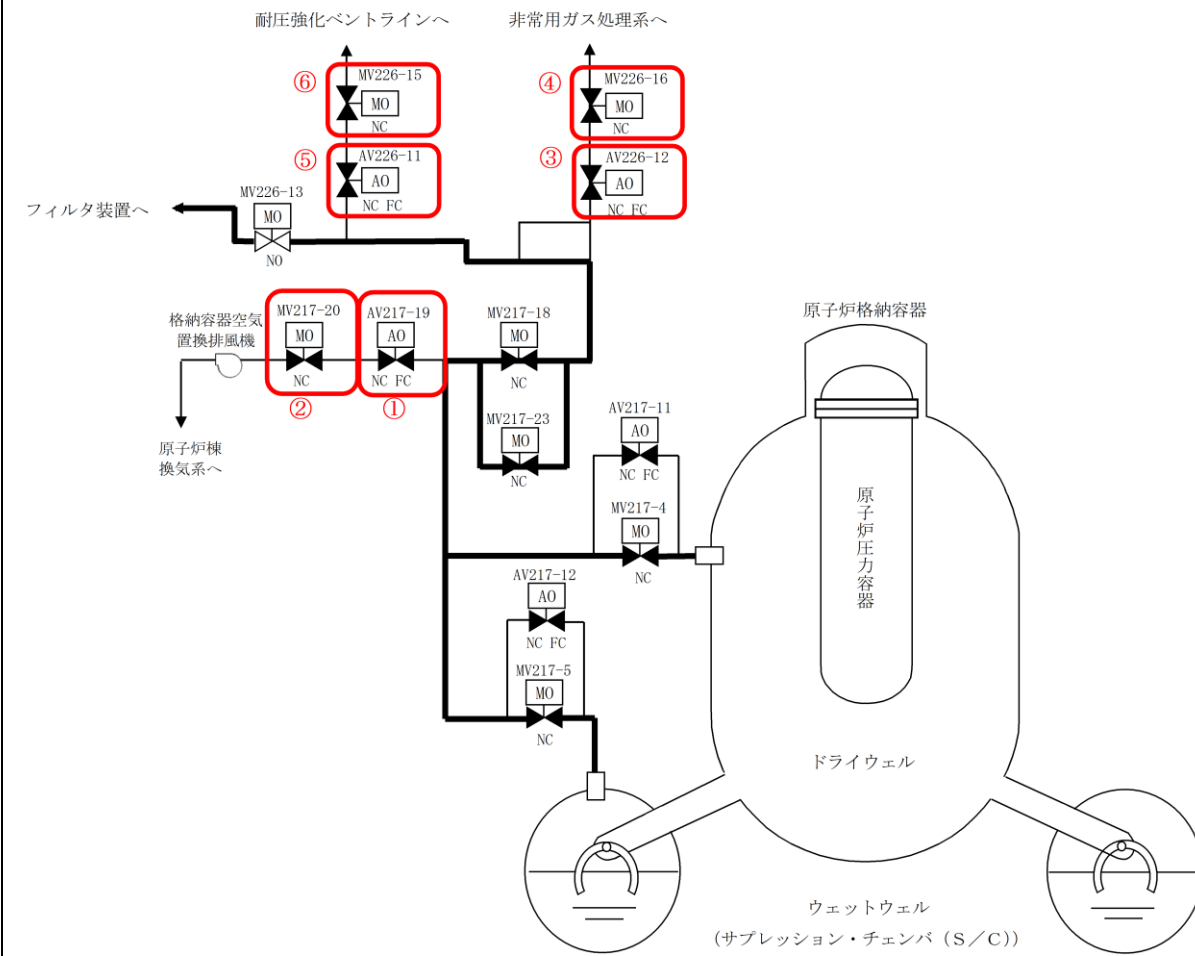
図9 他系統との隔離弁の概略構成図
